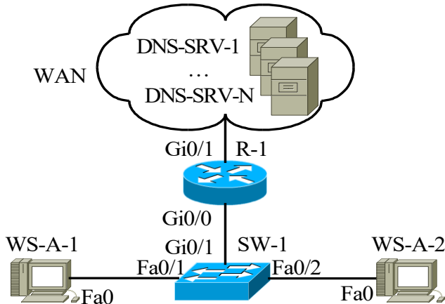
Рис. 7. Приклад мережі
