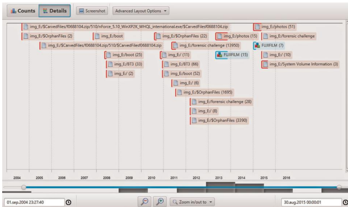
Рис. 53. Часова шкала в Autopsy
