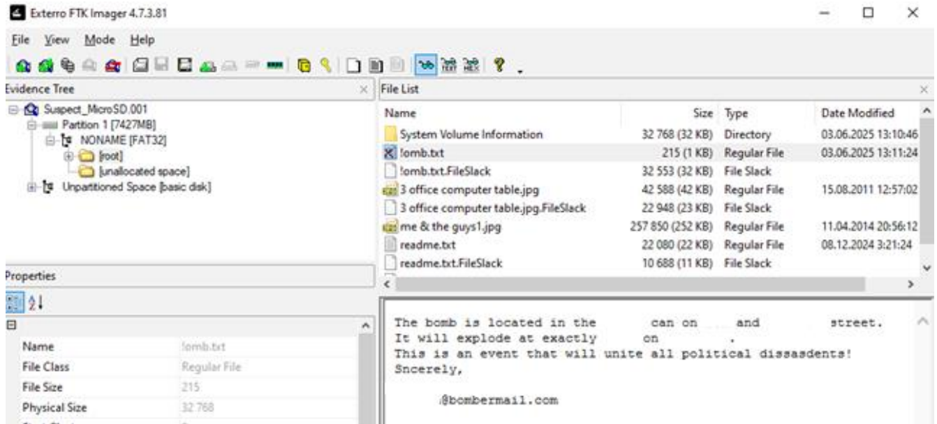
Рис. 31. Пошук видаленого файлу у FTK Imager
