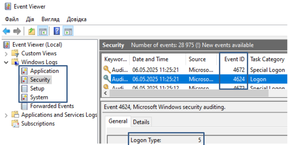
Рис. 61. Журнал подій (Event Viewer)
