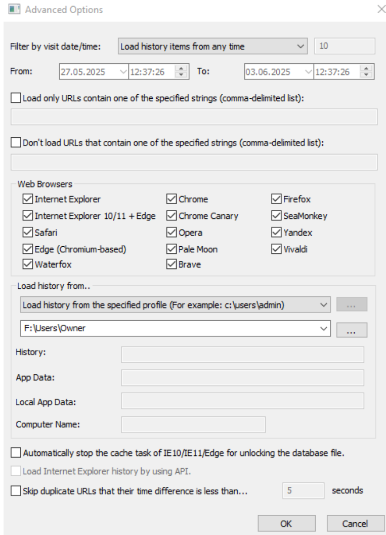
Рис. 108. BrowsingHistoryView
