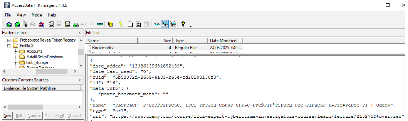
Рис. 100. Закладки
