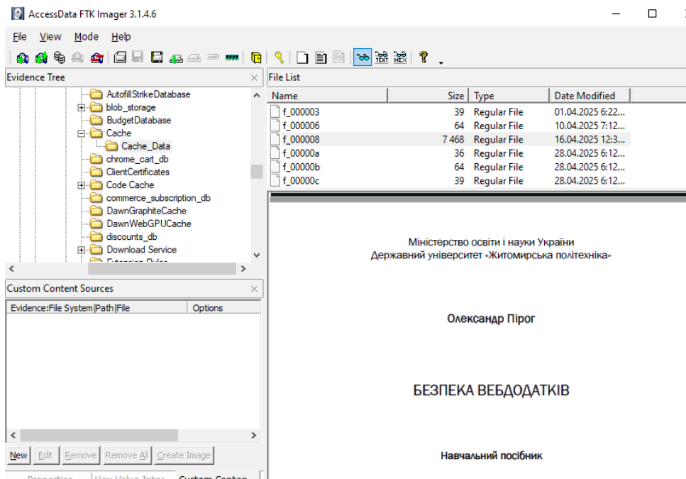
Рис. 98. Кеш браузера
