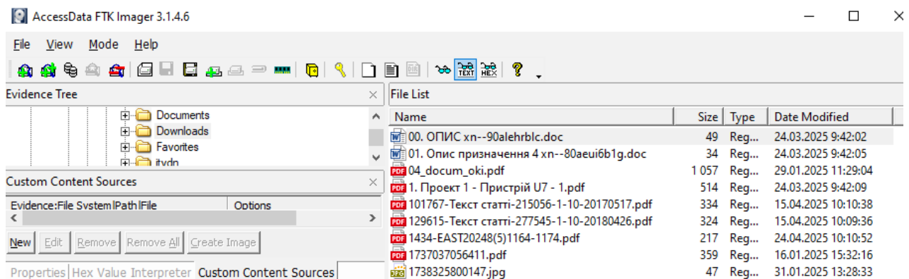
Рис. 101. Завантажені файли
