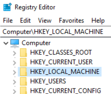
Рис. 64. Реєстр Windows
