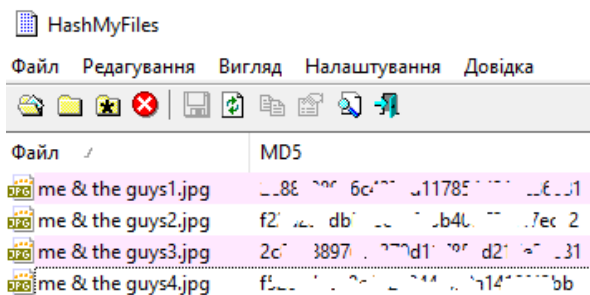
Рис. 8. HashMyFiles
