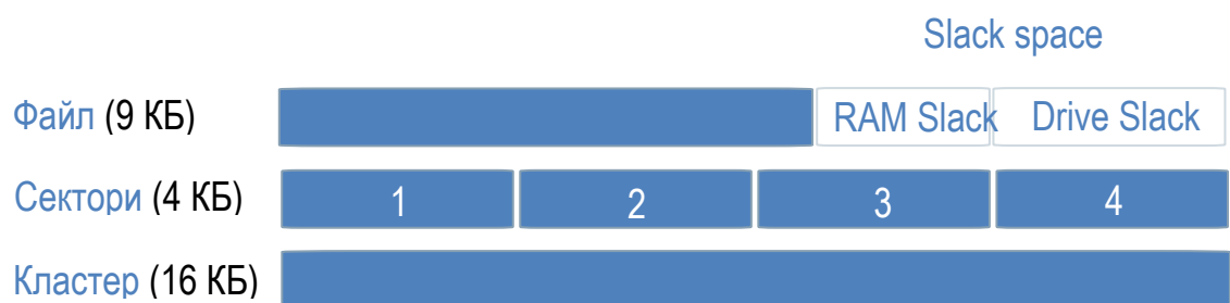
Рис. 21. Slack Space
