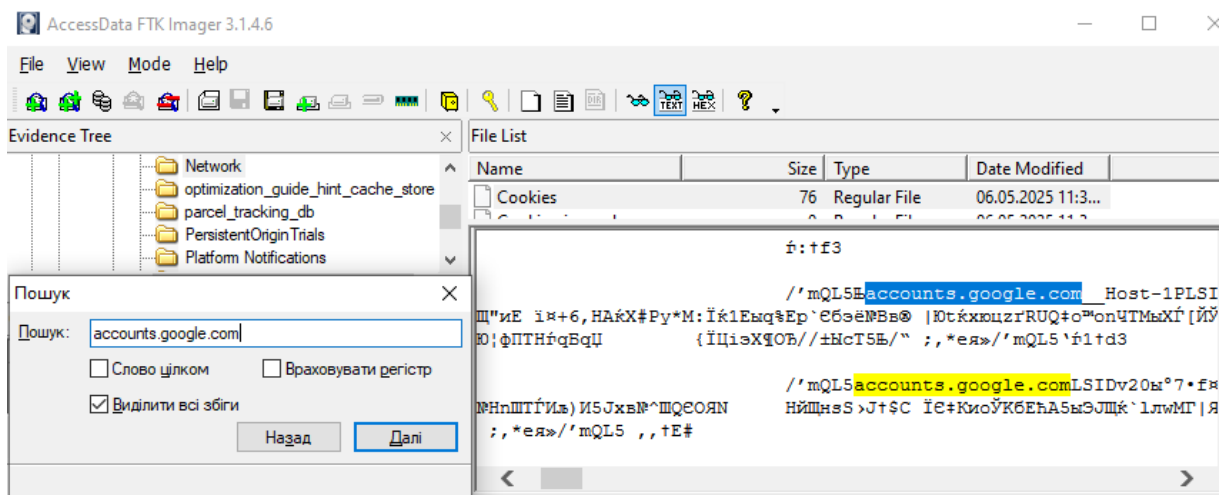
Рис. 99. Cookies
