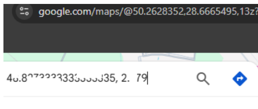
Рис. 56. Карти Google
