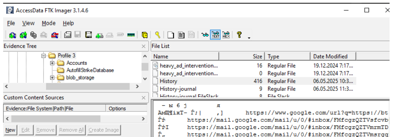
Рис. 97. Історія браузера
