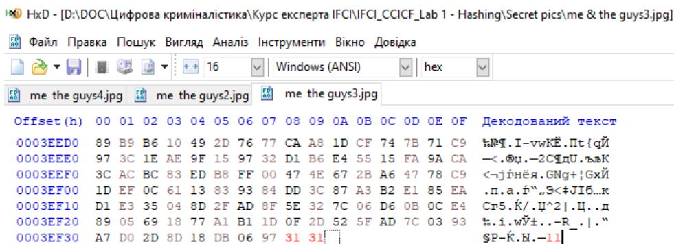
Рис. 9. HxD
