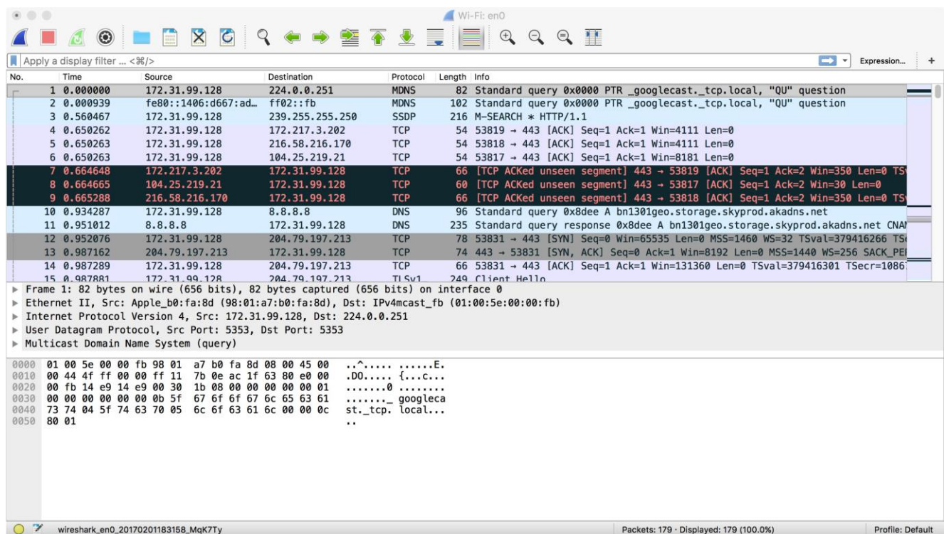
Рис. 107. Wireshark
