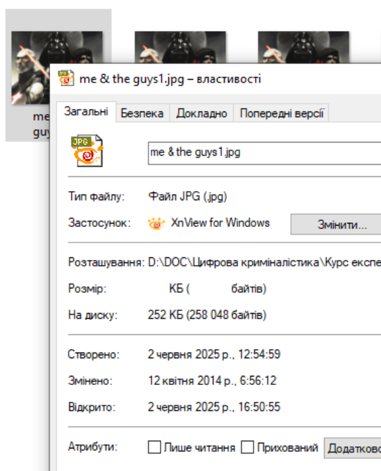
Рис. 7. Властивості файлу
