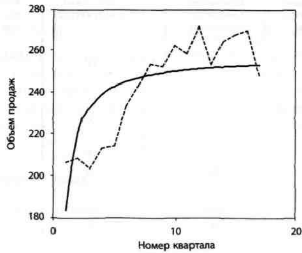
Рис. 7. Крива підгонки – гіпербола
