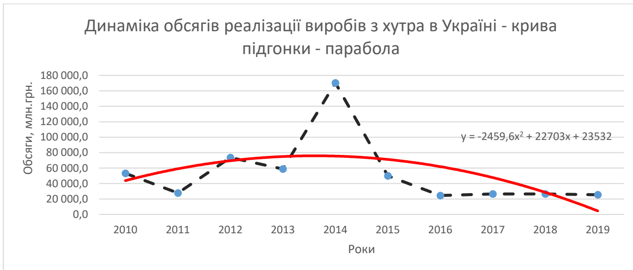
Рис. 2. Крива підгонки – парабола
