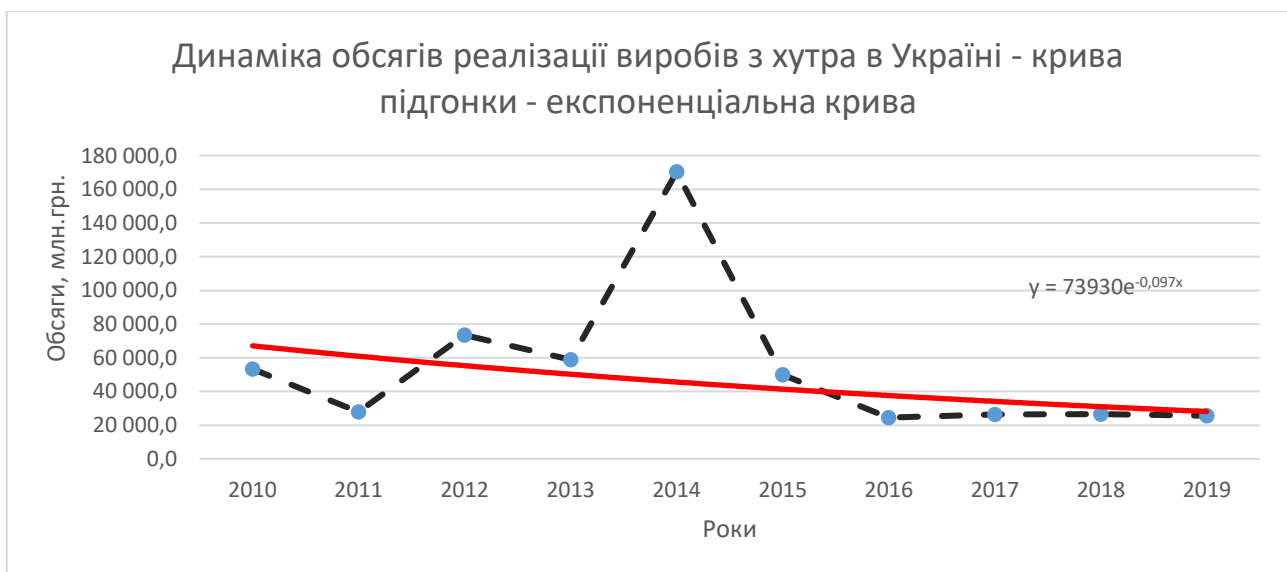
Рис. 5. Крива підгонки – експоненціальна крива
