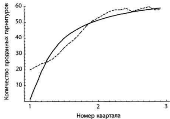
Рис. 8. Крива підгонки – S-образна крива
