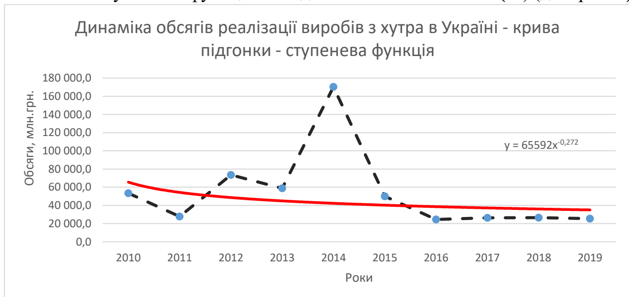
Рис. 6. Крива підгонки – графік ступеневої функції
