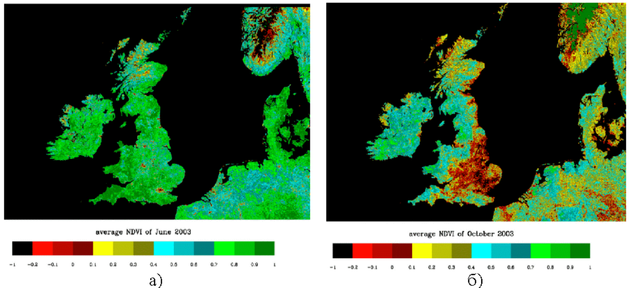
Рис. 2.37 – Змінення з часом індексу вегітації: а – зображення NDVI у червні; б – зображення NDVI у жовтні
