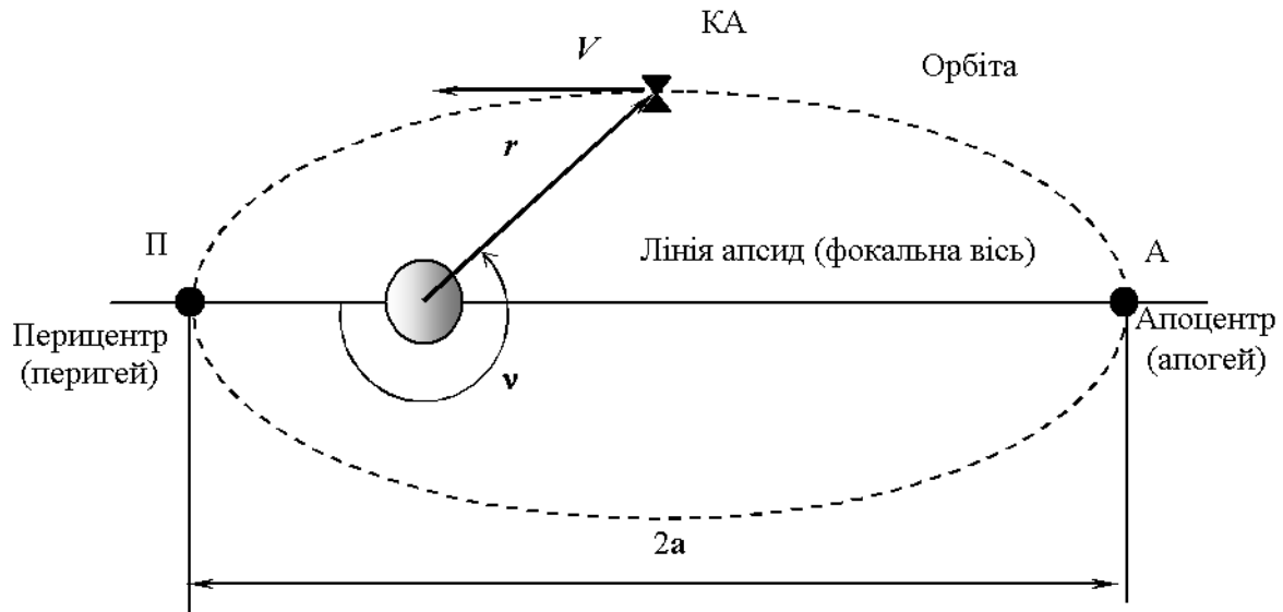
Рис. 1.13 – Орбіта КА (еліпс)
