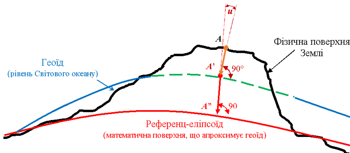
Рис. 2.18 – Проеціювання точки з поверхні Землі на геоїд та на референц-еліпсоїд
