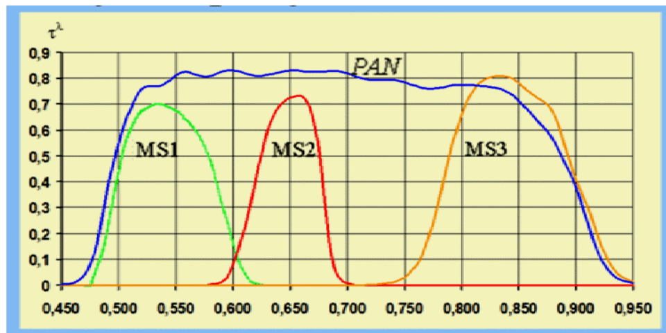
Рис. 1.31 – Зовнішній вигляд спектроподільного блоку (а) та смуги пропускання спектральних каналів МСУ-8 (б)
