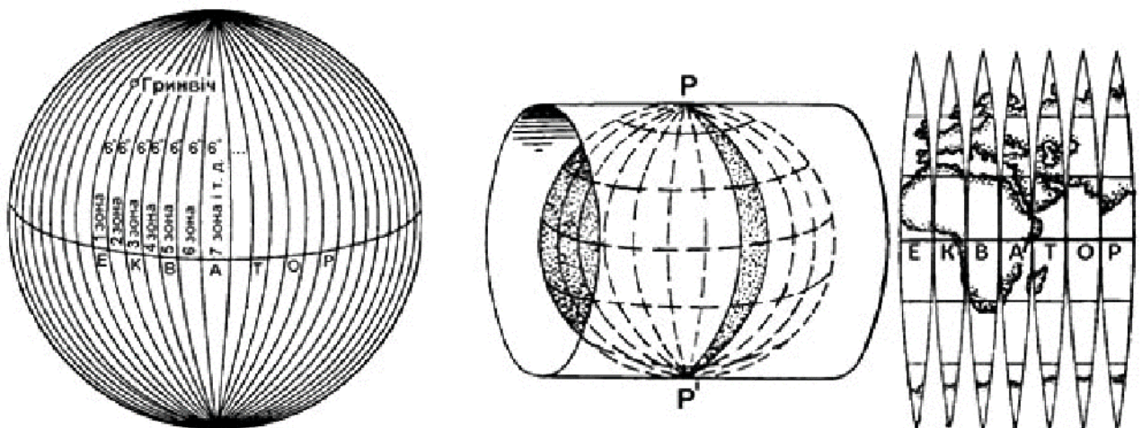
Рис. 2.23 – Поділення земного еліпсоїда на шість градусні зони
