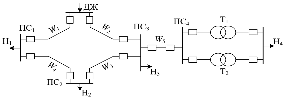
Рис. 1. Принципова схема мережі
