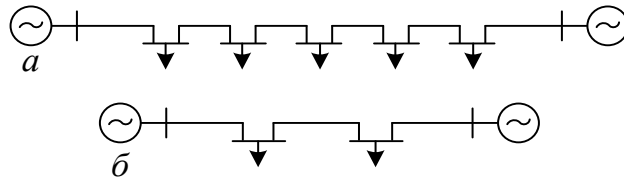
Рис. 6. Однотипні схеми з різним ступенем надійності
