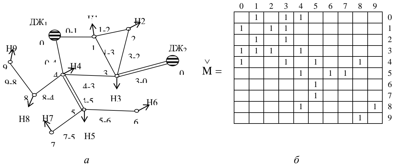
Рис. 4. Схема електричної мережі (а) та її матриця вузлів (б)
