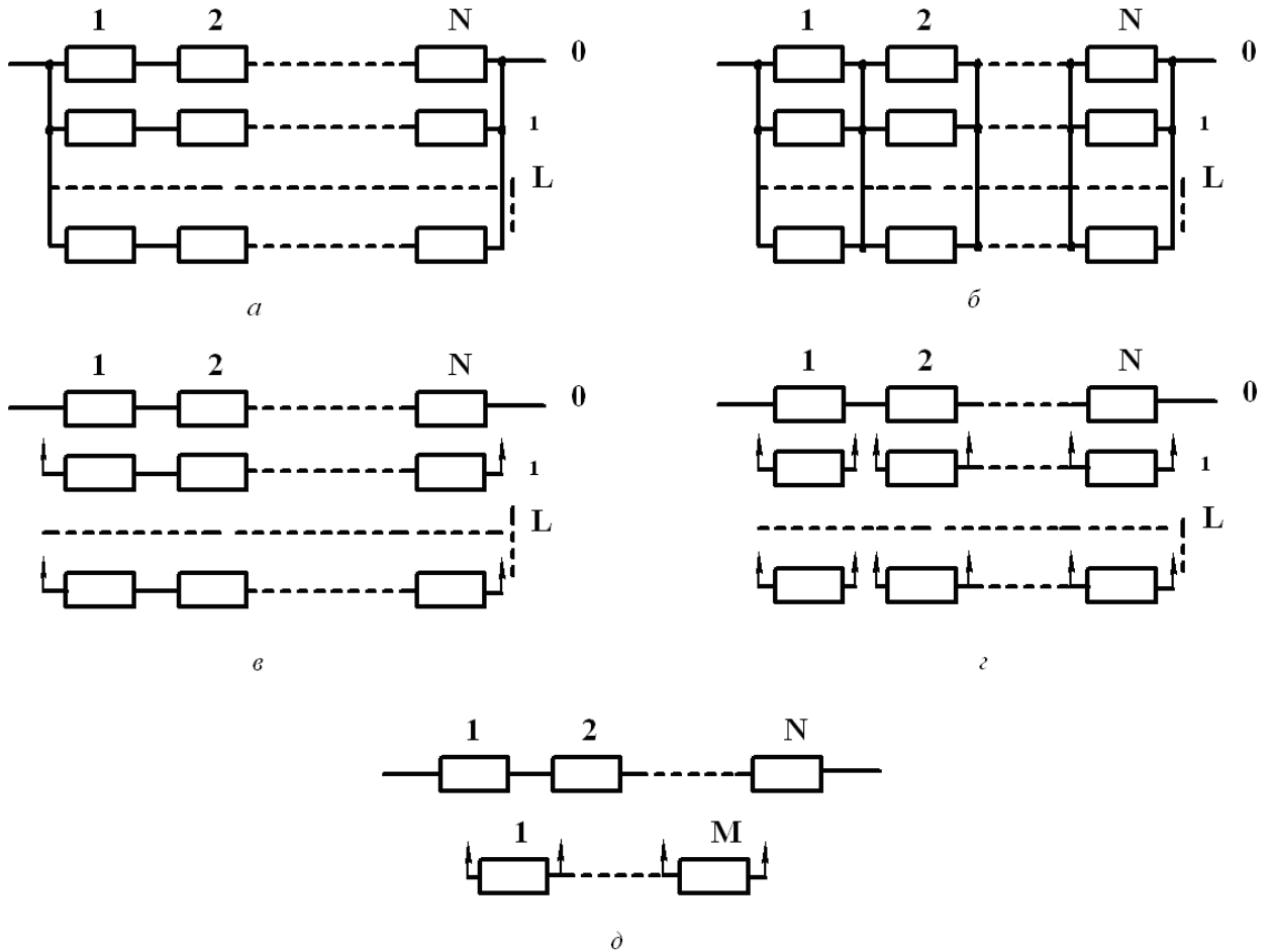
Рис.1. Схема резервування: a – загального постійного; б – поелементного постійного; в – загального заміщувального; г – поелементного заміщувального; д – ковзного
