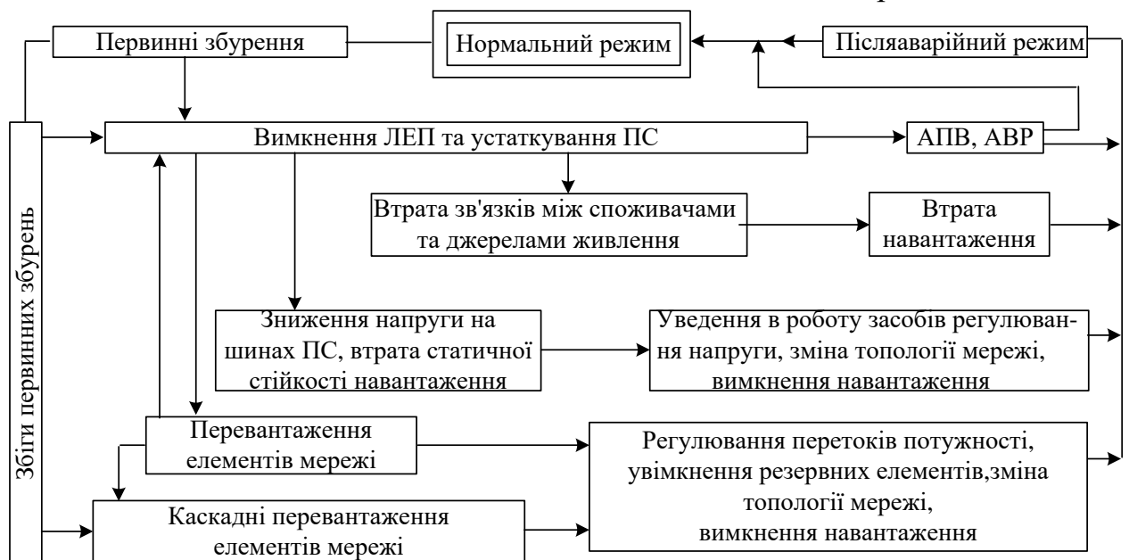
Рис. 5. Аварійні режими електричних мереж та їх ліквідація
