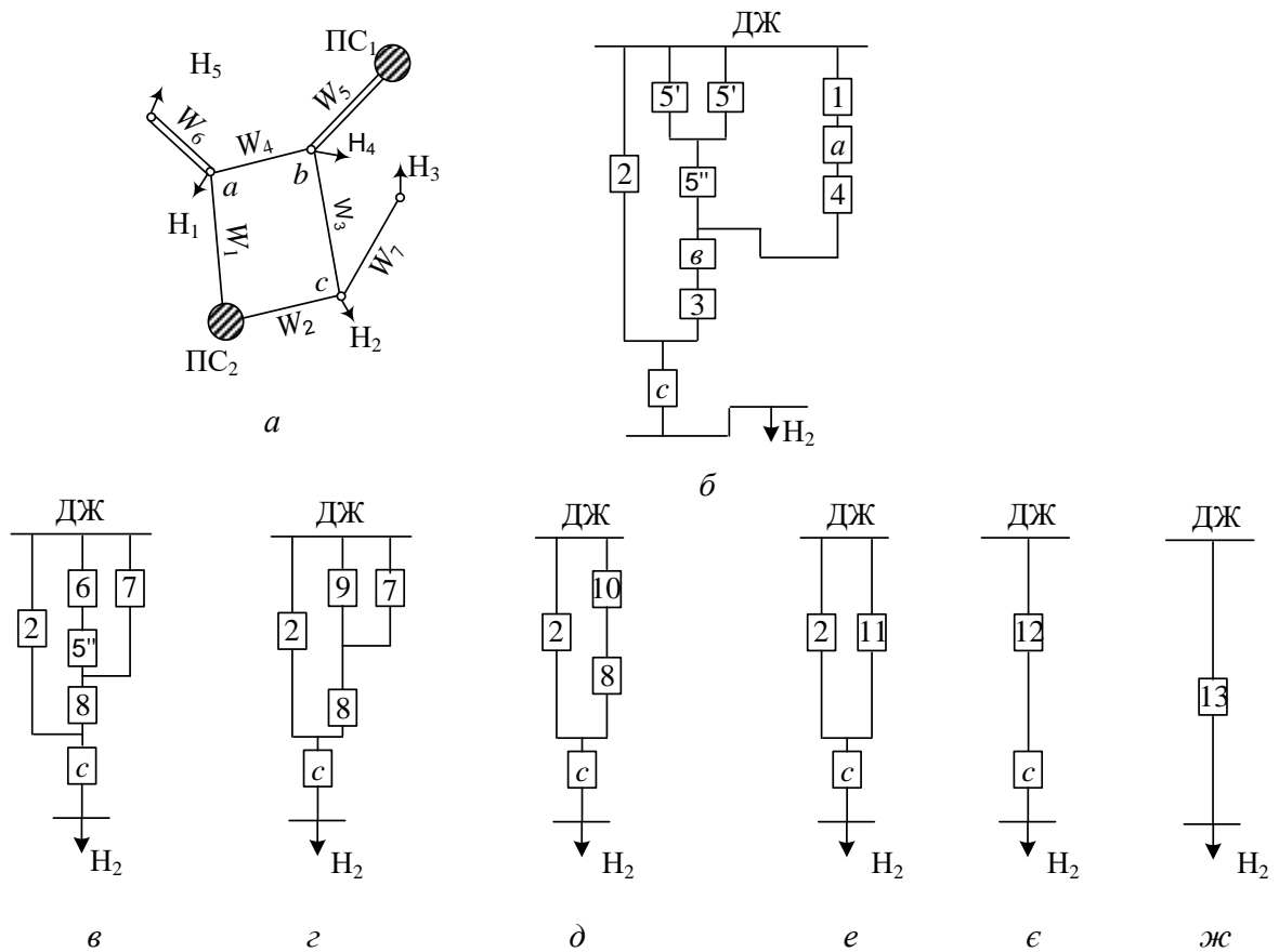
Рис. 2. Складання та етапи перетворення розрахункової схеми надійності
