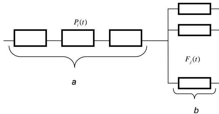
Рис. 5. Комбінована система з послідовним і паралельним з'єднанням елементів
