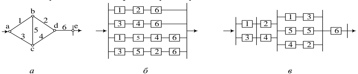
Рис. 3. Схема мережі (а) та її еквівалентні розрахункові схеми надійності (б,в)
