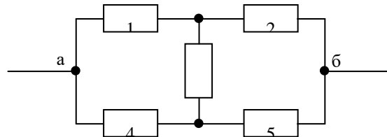
Рис. 5.11. Логічна схема складної системи для розрахунку надійності
