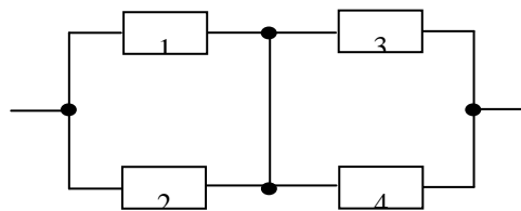
Рис 5.1. Паралельно-послідовне з'єднання елементів
