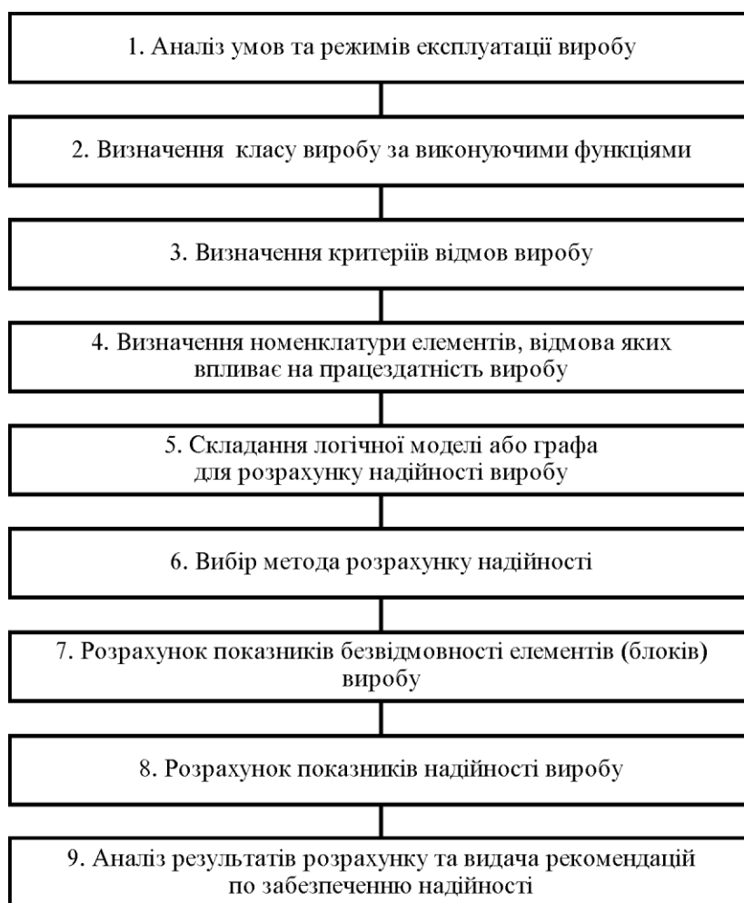
Рис. 6.1. Наближений алгоритм розрахунку надійності при проектуванні виробу
