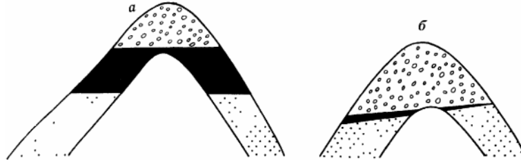
Рис. 12.3. Умови залягання газу, нафти і води в пастці
