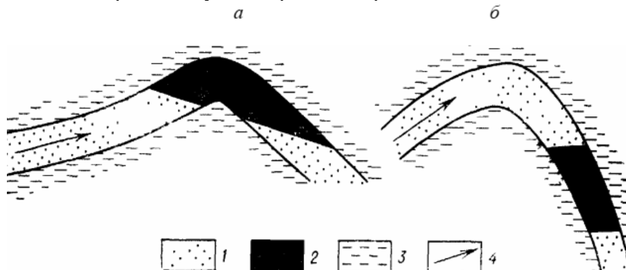
Рис. 12.4. Зміщення покладу нафти рухомими водами
