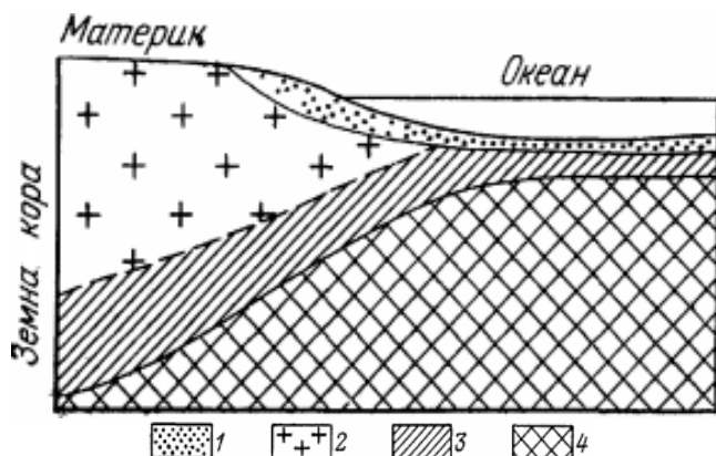
Рис. 2.4. Схема будови континентальної і океанічної кори
