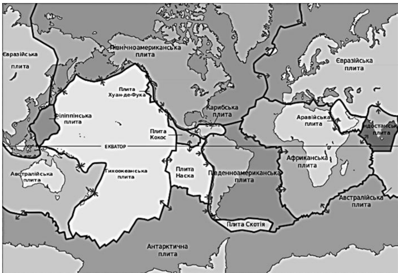
Рис. 5.10. Основні літосферні плити
