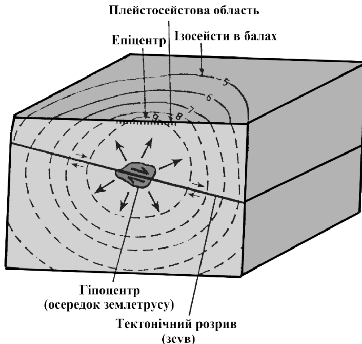
Рис. 5.8. Гіпоцентр та епіцентр землетрусу
