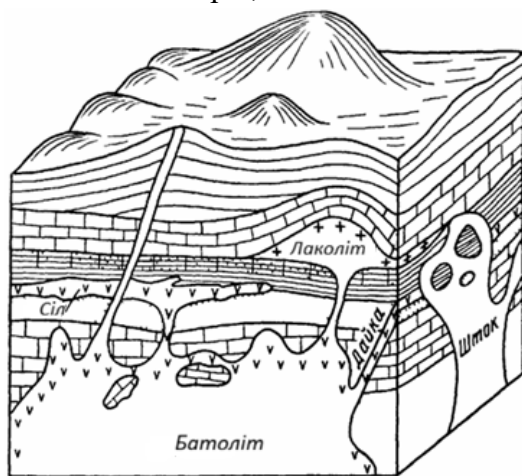
Рис. 5.1. Форми залягання інтрузій
