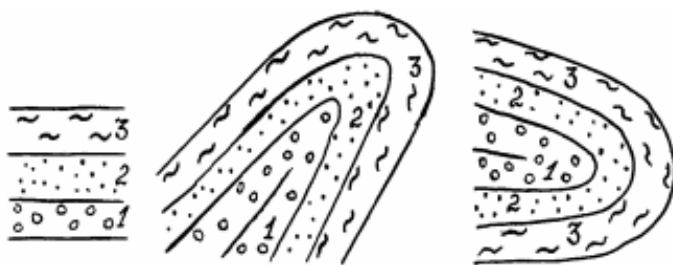
Рис. 4.4. Послідовність утворення геологічних тіл 1 – самий древній шар; 2 – проміжний шар; 3 – самий молодий шар
