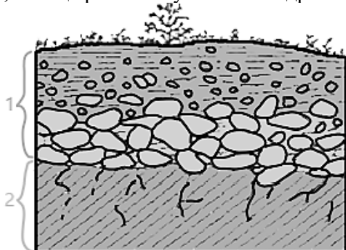
Рис. 6.1. Схема вивітрювання ґрунтових гірських порід
