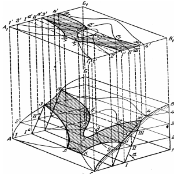
Рис. 10.3. Зображення на геологічній карті похило залягаючого пласта з крутим падінням
