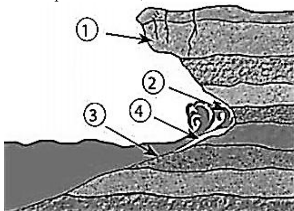
Рис. 6.6. Механізм абразійного процесу
