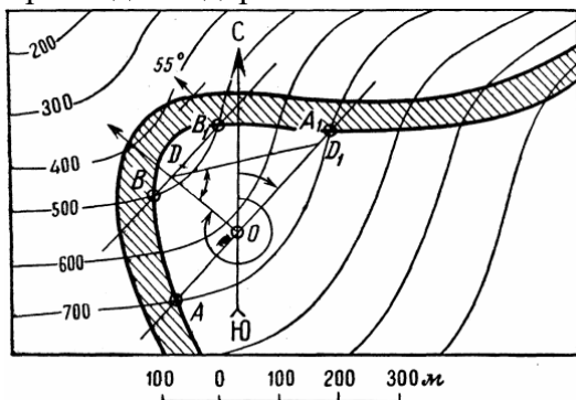
Рис. 10.4. Визначення елементів залягання пласта по геологічній карті AA 1 , BB 1 – лінії простягання пласта; кут COA 1 – азимут простягання пласта; OD – лінія падіння пласта; кут CD 1 OD – азимут падіння пласта; кут D 1 DO – кут падіння пласта
