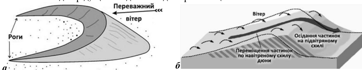
Рис. 6.2. Бархан (а) і дюна (б)
