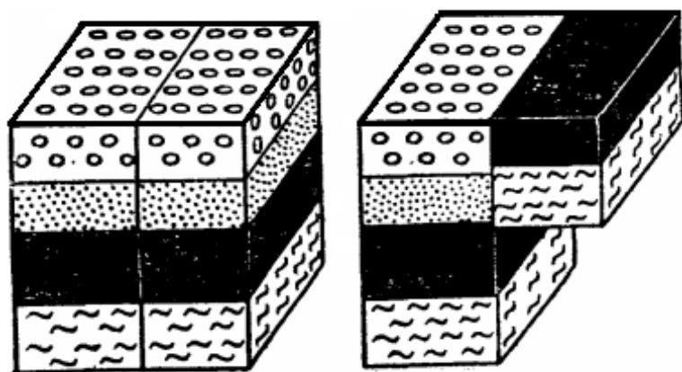
Рис. 10.7. Блок-діаграма, яка пояснює зображення скиду в горизонтально залягаючих пластах
