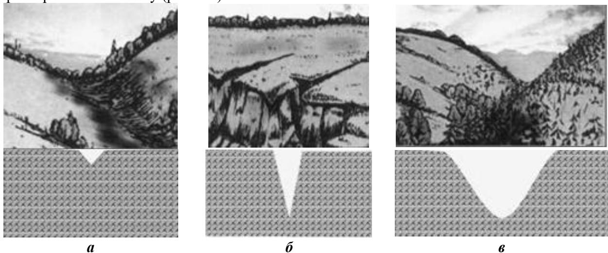
Рис. 3.4. Стадії розвитку яру
