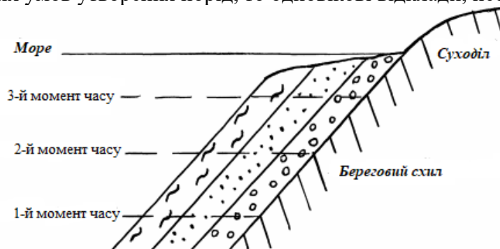
Рис. 4.5. Різновікові утворення геологічних шарів
