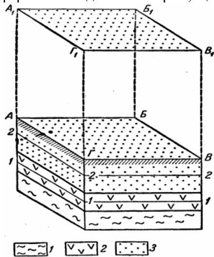
Рис. 10.1. Зображення на геологічній карті горизонтальне залягання пластів в умовах горизонтального рельєфу
