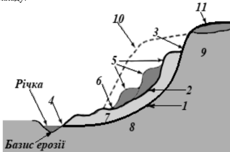
Рис. 11.2. Основні елементи зсувного цирку
