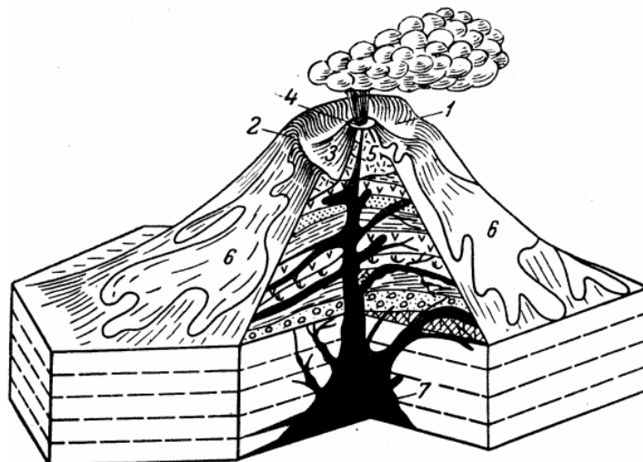
1 – кальдера; 2 – сома; 3 – конус; 4 – кратер; 5 – жерло; 6 – лавовий потік; 7 – лавовий осередок Рис. 5.2. Схема будови вулканічного апарату
