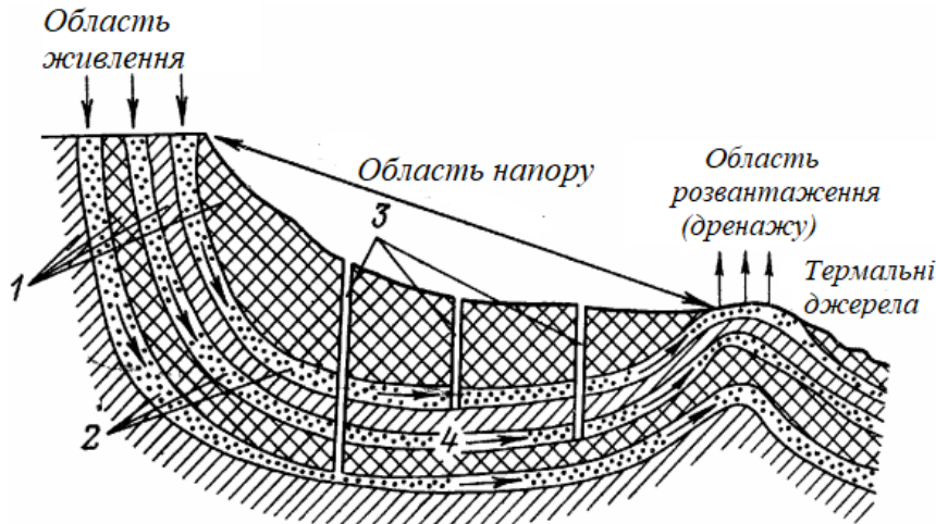
Рис. 12.2. Схема будови артезіанського басейну
