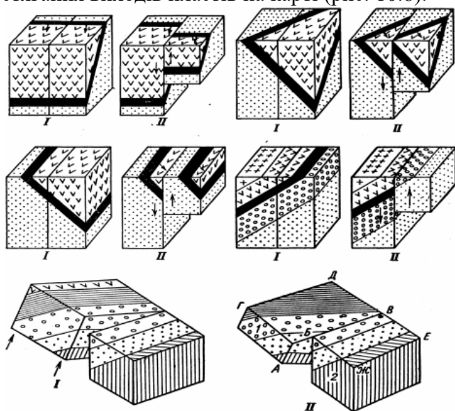
Рис. 10.8. Блок-діаграми, які пояснюють зображення скиду в похило залягаючих пластах на геологічній карті
