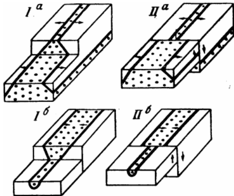
Рис. 10.9. Блок – діаграми, які пояснюють зображення на карті розривних порушень в умовах складчастого залягання порід I^a і I^б – положення до скиду; II^a і II^б – положення після скиду і розмиву піднятого крила
