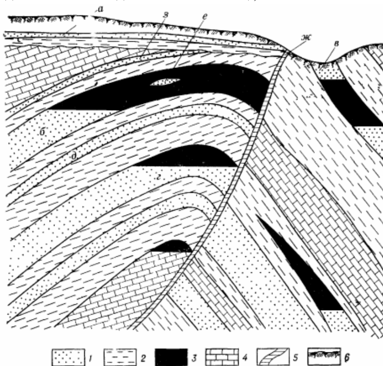
Рис. 12.5. Промислова класифікація підземних вод
