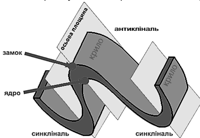
Рис. 5.6. Антиклінальна і синклінальна складки та їх елементи
