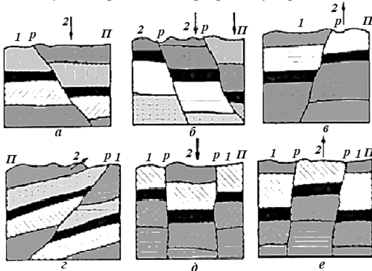
Рис. 5.7. Розривні дислокації:
