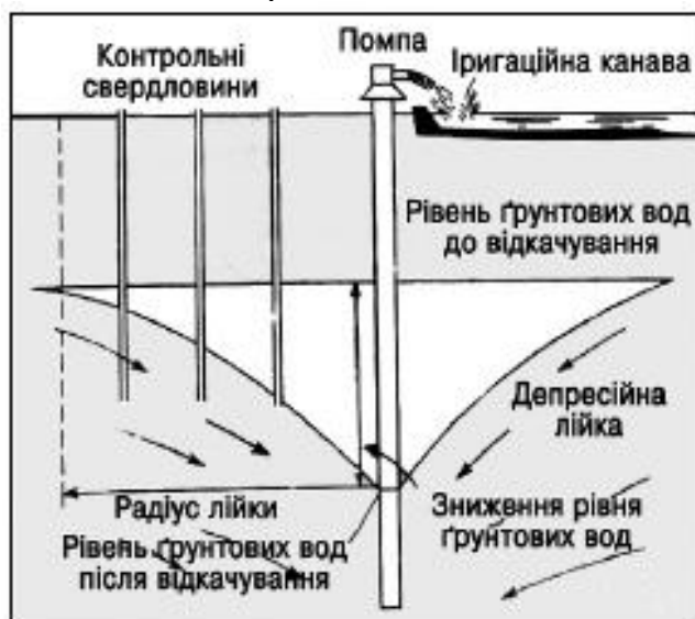
Рис. 12.1. Депресійна лійка в дзеркалі ґрунтових вод навколо свердловини
