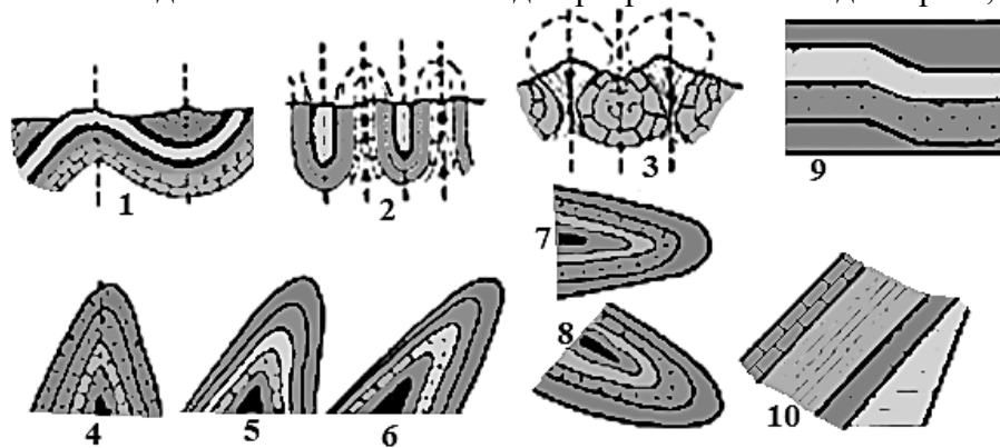
Рис. 5.5. Види складок
