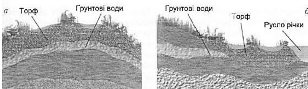
Рис. 6.7. Типи боліт
