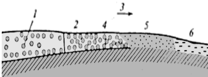
Рис. 5.9. Схема утворення флювіогляціальних відкладів:
