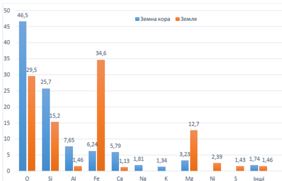
Рис. 2.6. Хімічний склад земної кори та Землі (гіпотетичний)
