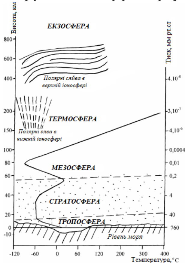
Рис. 2.5. Вертикальний розріз атмосфери
