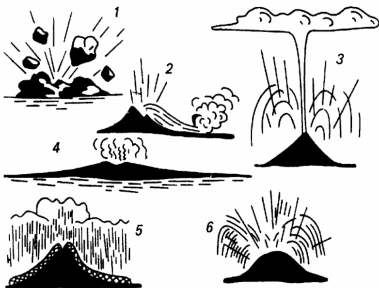
Рис. 5.3. Типи вивержень вулканів
