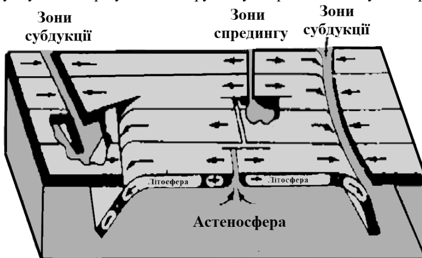
Рис. 5.9. Динаміка зародження (спредингу) і поглинання (субдукції) літосфери
