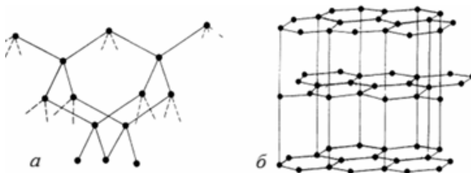
Рис. 3.1. Приклади кристалічних ґраток мінералів а – алмаз; б – графіт
