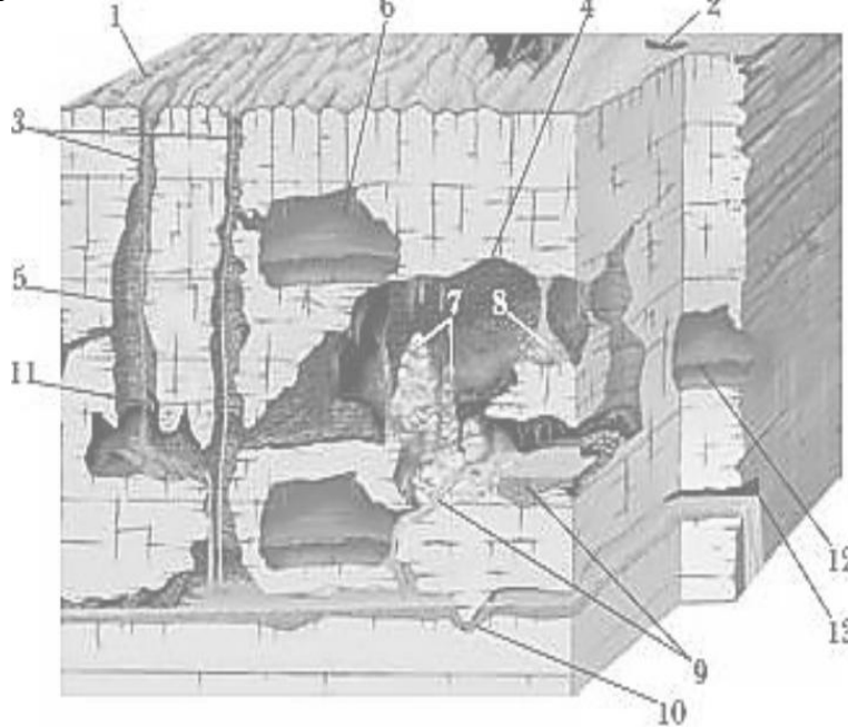
Рис. 11.1. Схема карстових процесів у гірському масиві
