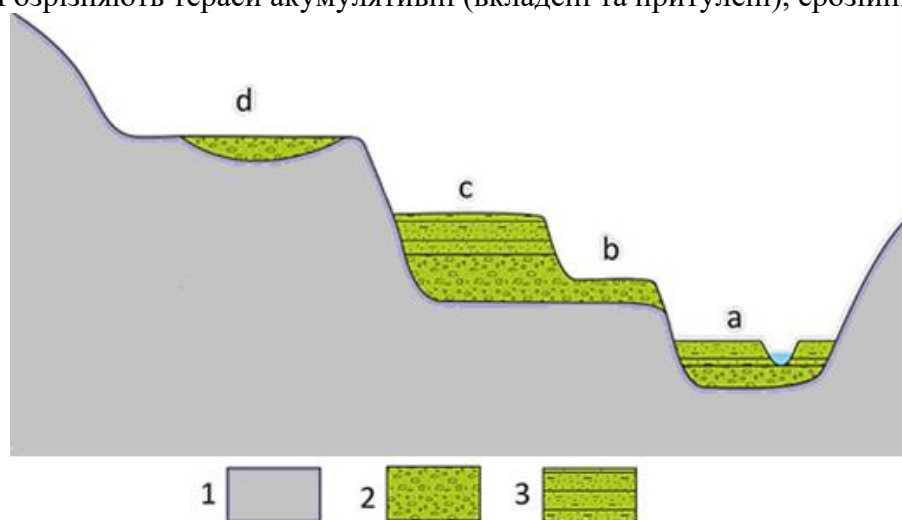
Рис. 6.5. Приклади генетичних видів річкових терас a – заплава; b – цокольна (перша надзаплатна) тераса; c – аккумулятивна (друга надзаплатна) тераса; d – ерозійна (третья надзаплатна) тераса; 1 – корінні породи; 2 – русловий алювій; 3 – заплатний алювій
