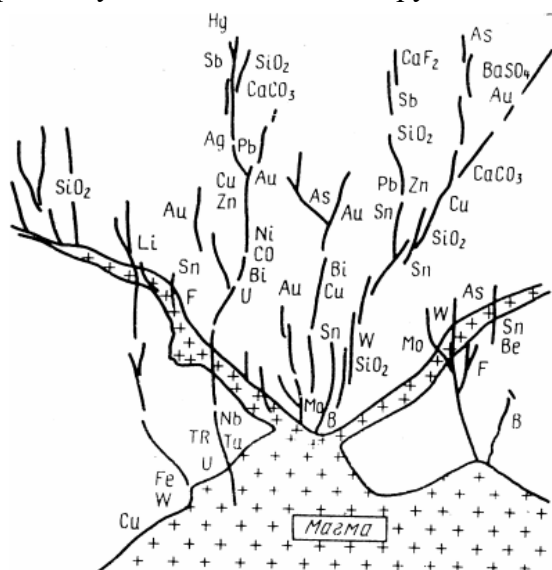
Рис. 5.4. Зональність зруденіння відносно магматичного осередку
