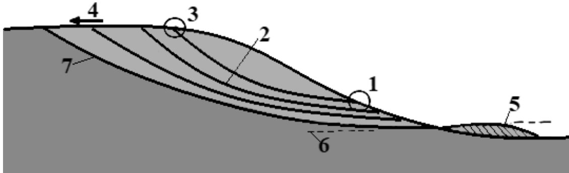
Рис. 6.3. Поздовжній профіль яру
