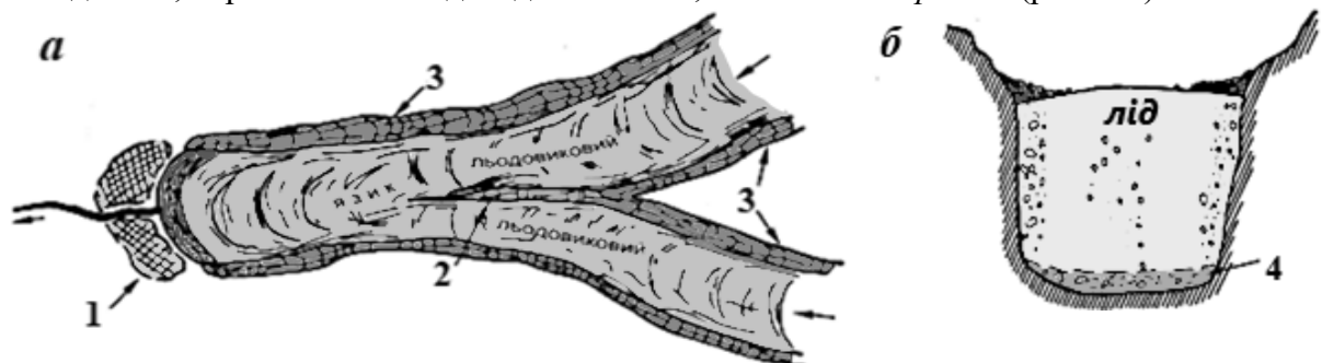
Рис. 6.8. Морени гірського льодовика
