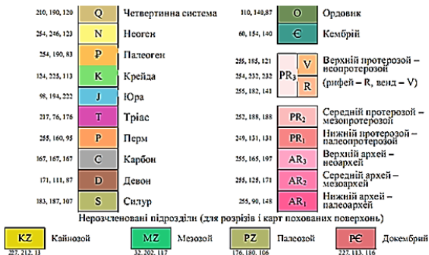
Рис. 1.4. Основні кольори розфарбовування стратиграфічних підрозділів
