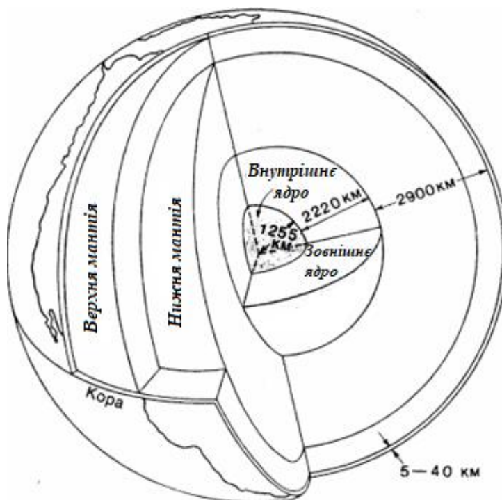
Рис. 2.2. Внутрішня будова Землі
