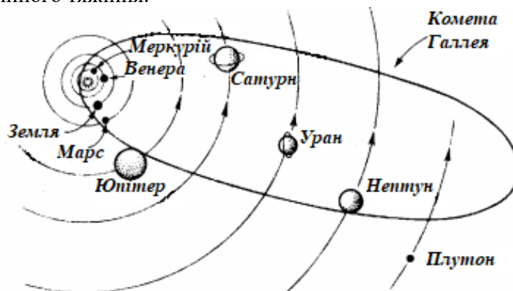
Рис.2.1. Будова Сонячної системи
