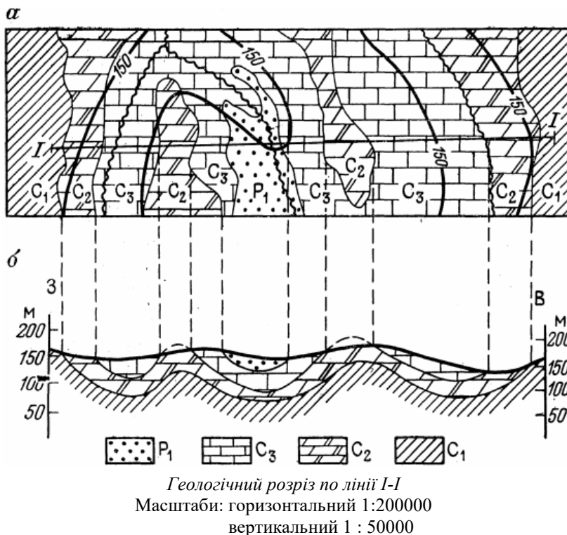
Рис. 10.10. Принцип побудови геологічного розрізу по геологічній карті: P_1 – нижній відділ пермської системи; C_3 – верхній відділ кам'яновугільної системи; C_2 – середній відділ кам'яновугільної системи; C_1 – нижній відділ кам'яновугільної системи
