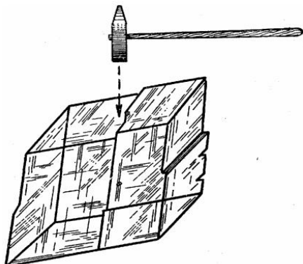
Рис. 3.6. Визначення напрямку спайності в кальциту
