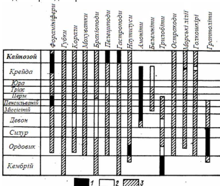
Рис. 4.2. Відносне хроностратиграфічне значення основних груп морських безхребетних протягом геологічного часу Групи: 1 – важливі для планетарних хроностратиграфічних кореляцій; 2 – застосовуються для регіональних кореляцій, 3 – іноді використовуються для місцевих кореляцій.
