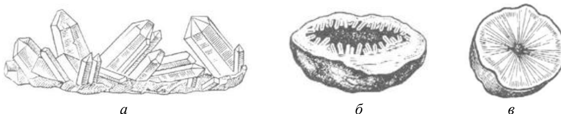
Рис. 3.5. Мінеральні агрегати: а – друза; б – секреція; в – конкреція
