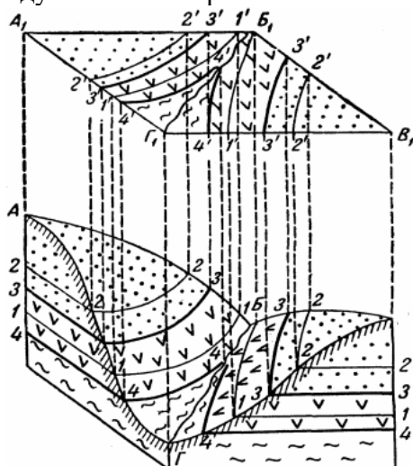
Рис. 10.2. Зображення на геологічній карті горизонтально залягаючих пластів в умовах перетнутого рельєфу
