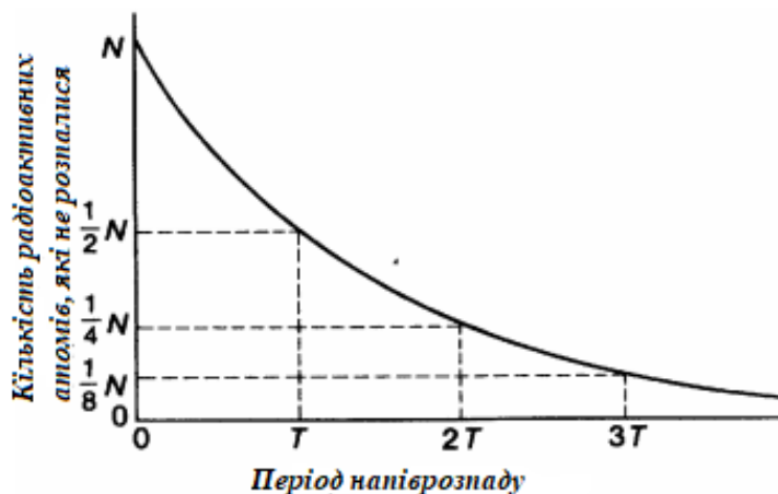
Періоди напіврозпаду радіоактивних елементів
