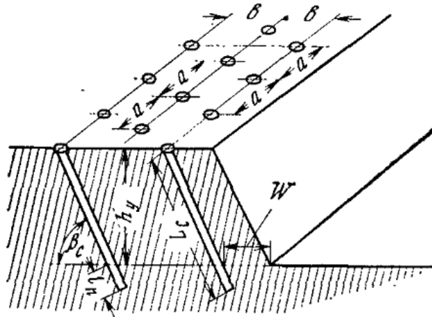
Рис. 2.2. Схема розташування свердловин на уступі
