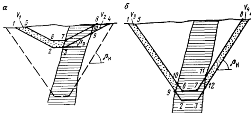
Рис. 1.3. Схема до визначення поточного (а) і контурного (б) коефіцієнту розкриву
