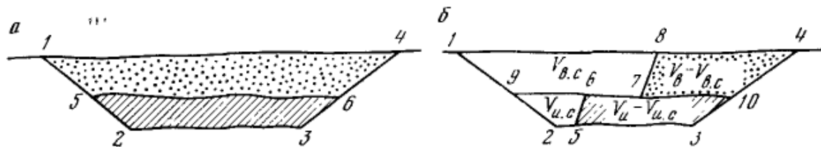
Рис. 1.2. Схема до визначення середнього геологічного (а) і середнього експлуатаційного (б) коефіцієнту розкриву: 1-5-6-4 – об’єм розкриву в кінцевих контурах кар’єру V_p , 5-2-3-6 – об’єм корисної копалини в кінцевих контурах кар’єру V_k , 1-9-10-4 – об’єм розкриву в кінцевих контурах кар’єру V_p , 1-9-7-8 – об’єм будівельного розкриву V_{pб} , 9-2-5-6 – об’єм корисної копалини видобутої при будівництві кар’єру (попутний видобуток) V_{кб}
