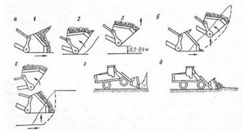
Рис. 3.23. Способи виймання порід навантажувачами
