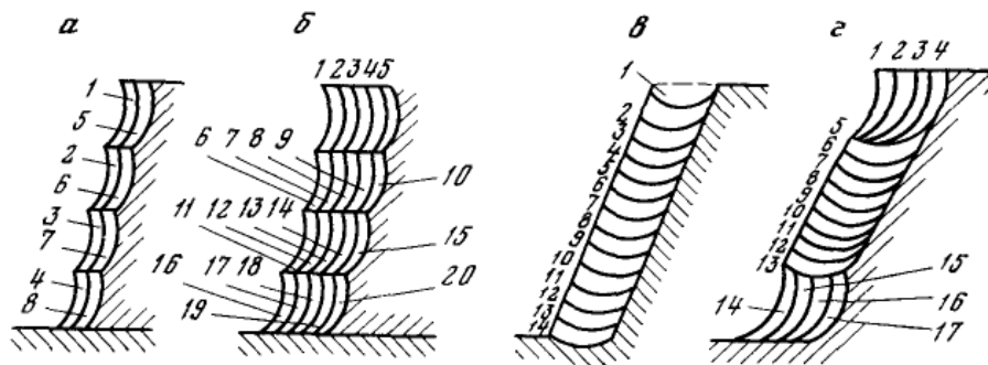
Рис. 3.20. Схеми виймання гірничої маси роторними екскаваторами: а – вертикальними поодинокими стружками; б – вертикальними багаторядними стружками; в – горизонтальними стружками; г – комбінацією вертикальних і горизонтальних стружок
