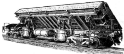
Рис. 4.4. Вагони-думпкари: а) в транспортному положенні; б) при розвантаженні
