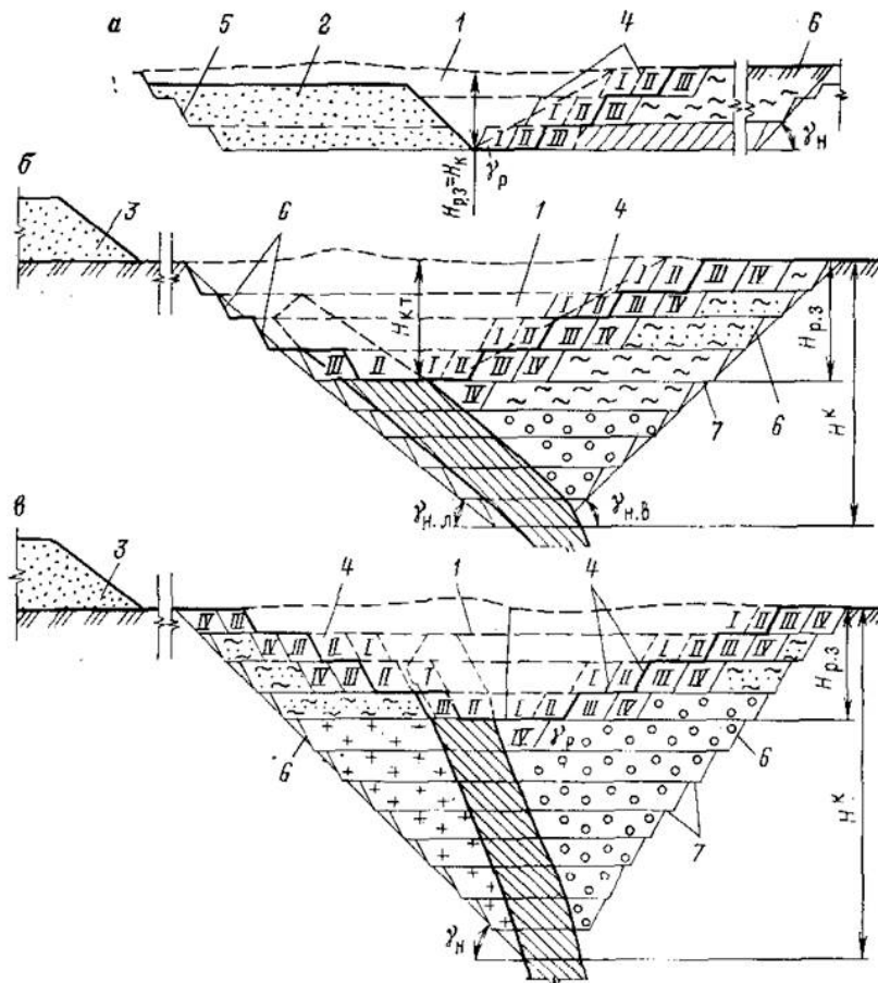
Рис. 1.1. Принципові схеми відкритої розробки покладав: а – горизонтальних; б – похилих; в – крутопадаючих; 1 – вироблений простір; 2, 3 – внутрішні і зовнішні відвали; 4, 5 – робочий і неробочий борти; 6 – кінцевий контур кар'єру; 7 – берми; I, II... – послідовність розвитку робіт на уступах
