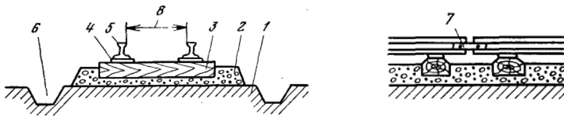
Рис. 4.6. Схема будови залізничного шляху: 1 – земельне полотно; 2 – баласт; 3 – шпала; 4 – підкладка; 5 – рейки; 6 – водовідводна канава; 7 – накладка; 8 – ширина колії
