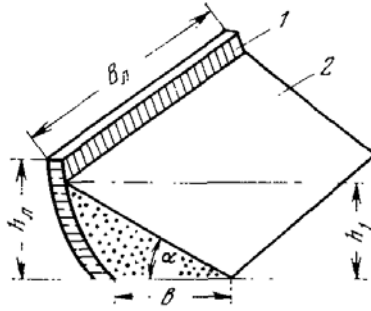
Рис. 3.21. Схема до визначення об'єму призми волочіння: 1 – відвал; 2 – гірнича маса
