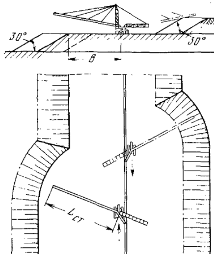
Рис.5.7. Схема відсіпки відвалу консольним відвалоутворювачем
