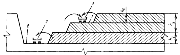
Рис. 1.12. Поперечний переріз кар'єру: 1 – робоча площадка верхнього уступу; 2 – робоча площадка нижнього уступу; 3 – транспортні засоби
