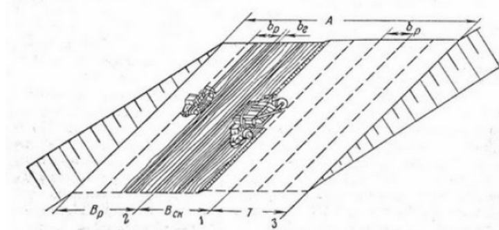
Рис.3.22. Торцевий скреперний забій: 1, 2, 3 – смуги скреперування, рихлення і транспортування
