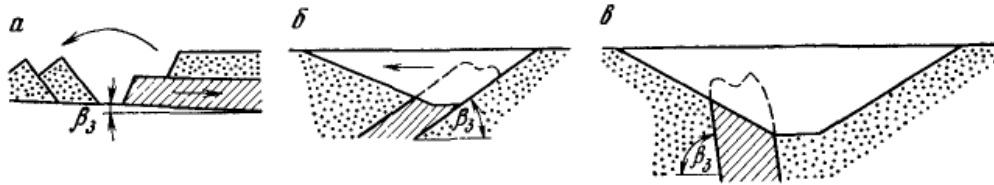
Рис. 1.14. Схеми поперечного перерізу кар'єру під час розробки відповідно пологого, похилого і крутого покладу
