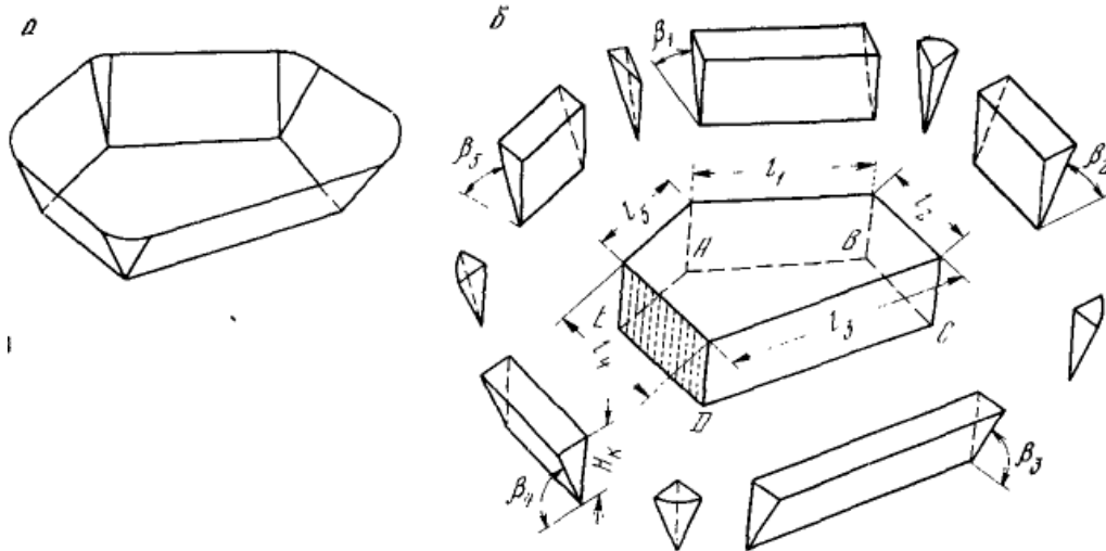
Рис. 1.6. Схема до визначення об'єму гірничої маси V_{\text{гм}} в контурах кар'єру: а – загальний вигляд; б – геометричні тіла, з яких складається об'єм кар'єру.
