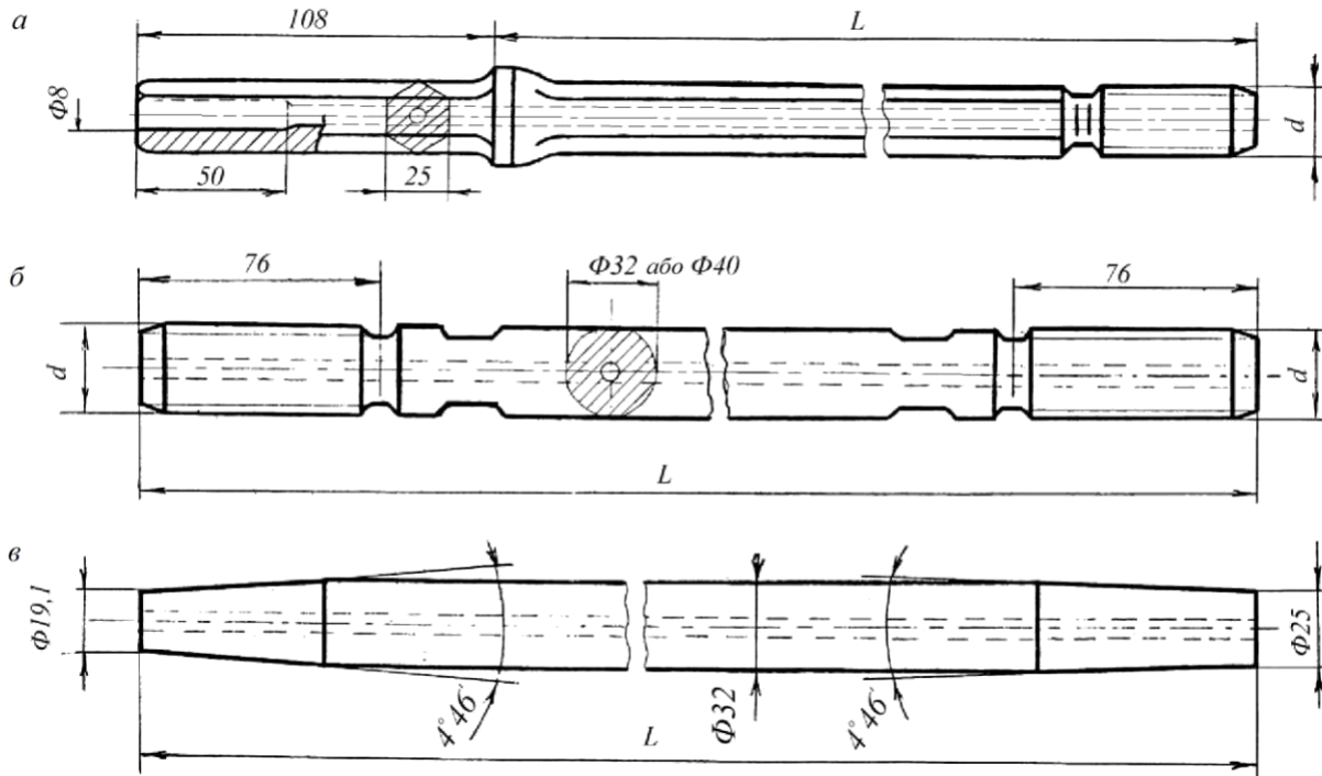
Рис. 21. Штанги (бури) перфраторів і бурильних головок
