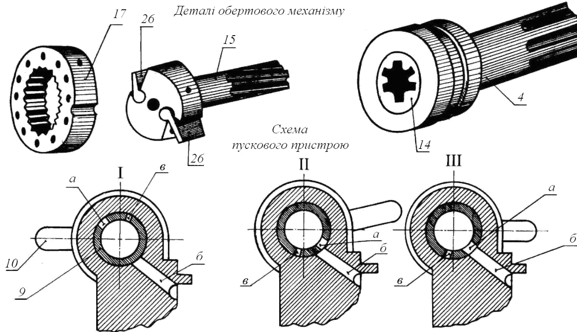
Рис. 4. Вузли перфоратора
