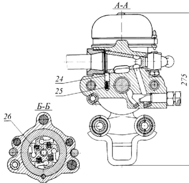
Рис. 14. Розрізи перфоратора із золотниковим повітророзподіленням типу ПП63СВП
