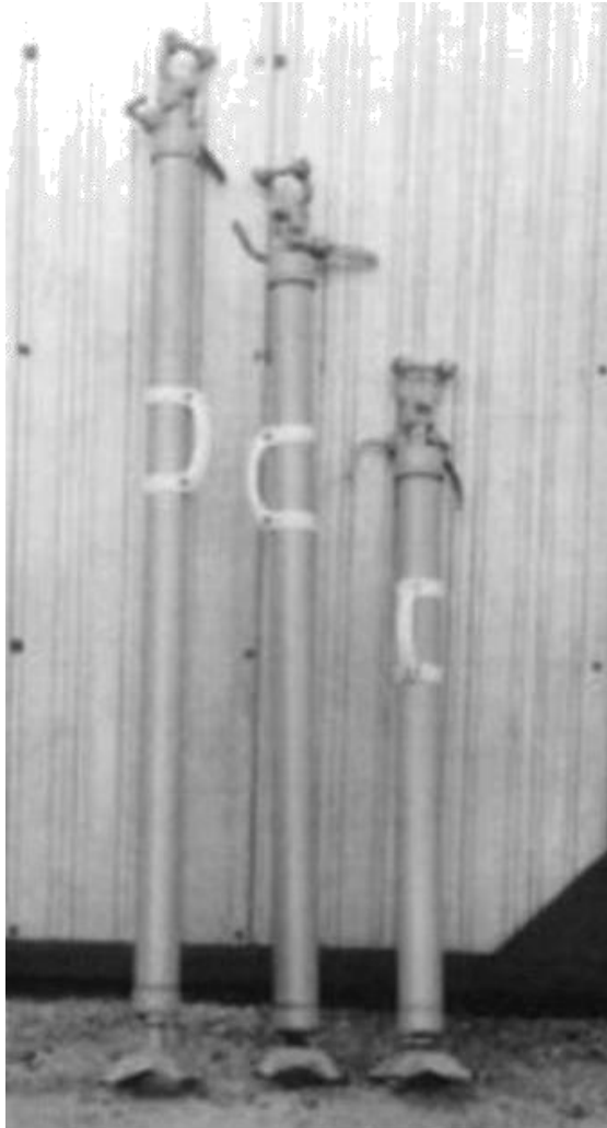
Рис. 24. Зовнішній вигляд пневмопідтримок П8, П11, П13
