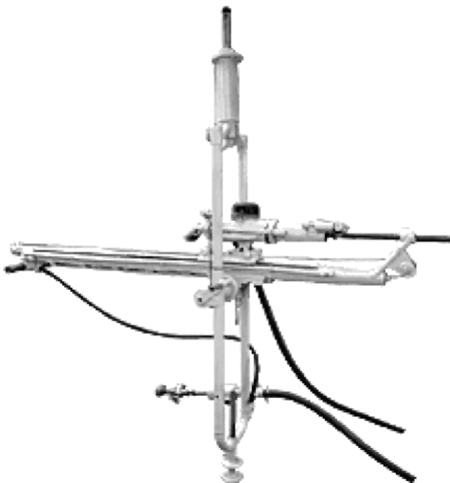
Рис. 26. Установка бурильна телескопічна універсальна УБТУ-1
