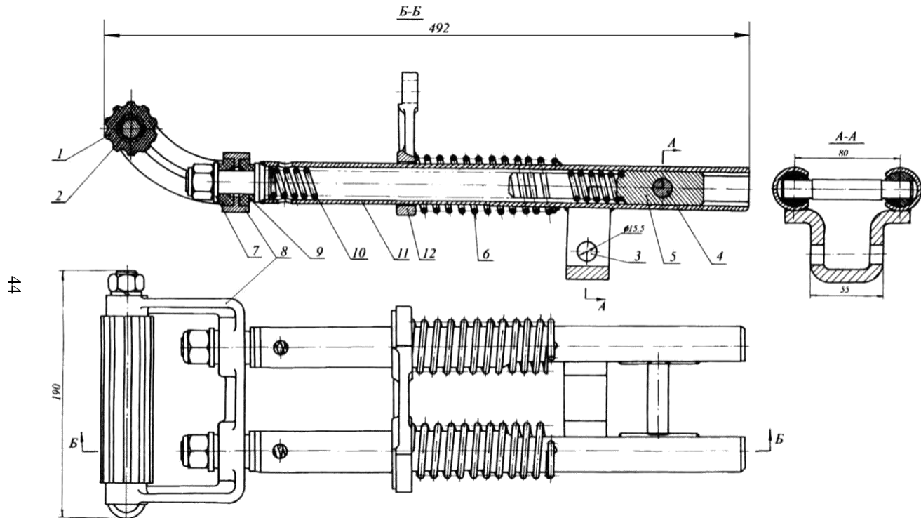
Рис. 17. Віброгасильна каретка типа КВУ1
