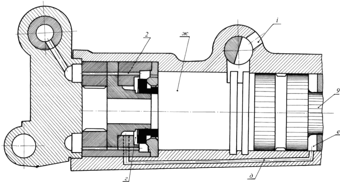
Рис. 11. Клапаний повітророзподільний пристрій (холостий хід)
