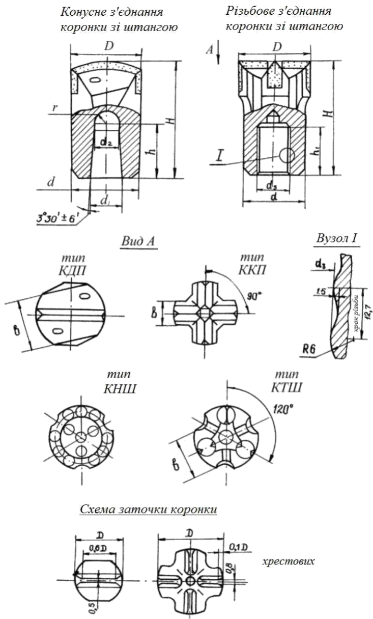
Рис. 22. Бурові коронки
