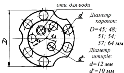
Чотириперова коронка
