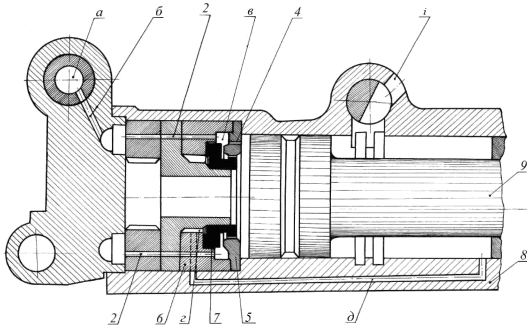
Рис. 10. Клапанний повітророзподільний пристрій (робочий хід)
