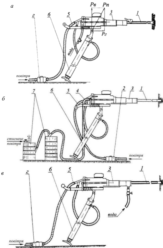
Рис. 15. Схеми монтажу переносного перфоратора з різними пристроями очищення шпуру від бурового пилу
