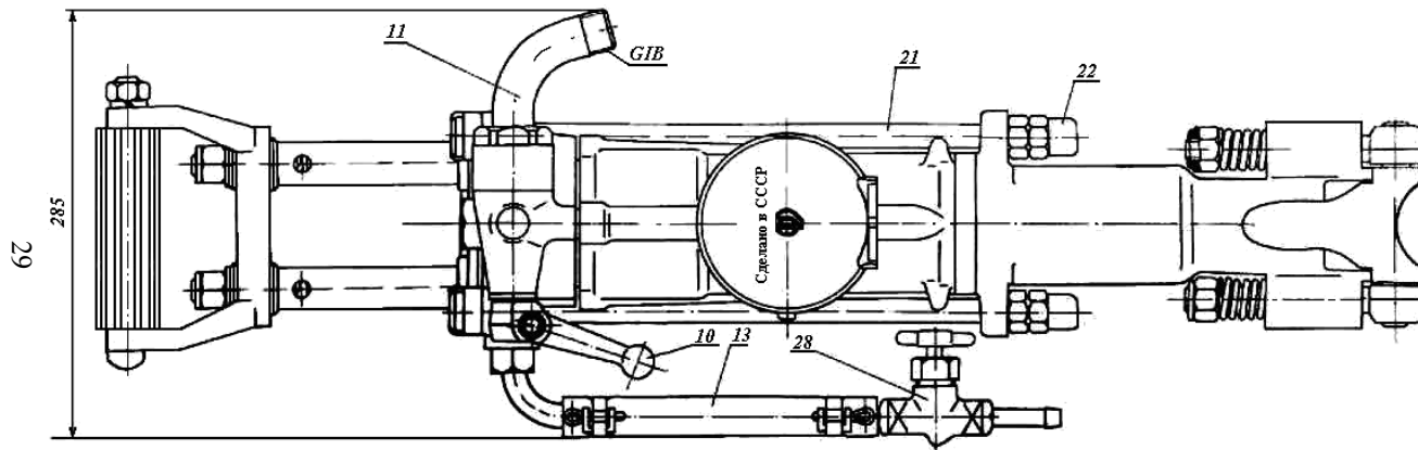
Рис. 2. Вигляд зверху переносного пневматичного перфоратора з центральним промиванням типу ПП63В
