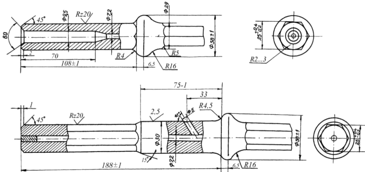
Рис. 19. Хвостовики шестигранных бурів з центральною і бічною подачею води для промивання
