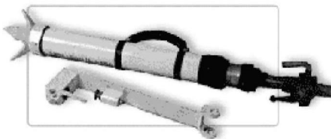
Рис. 27. Установка переносна бурильна УПБ-1Б
