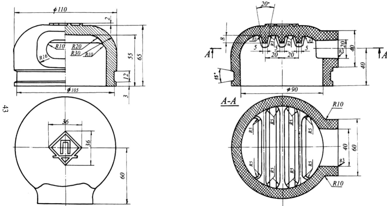
Рис. 16. Глушник шуму конструкції заводу "Пневматика"
