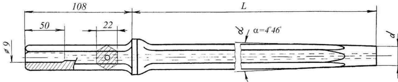
Рис. 20. Бури (штанги) переносних перфтораторів
