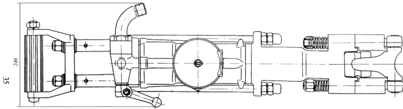
Рис. 8. Вигляд зверху переносного пневматичного перфоратора з бічним промиванням типу ПП63ВБ
