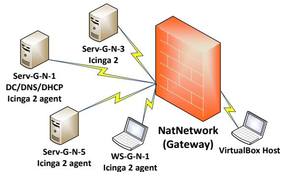
Рис. 6.1. Топологія мережі
