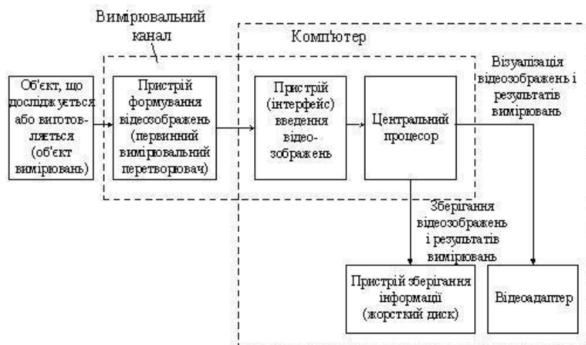
Рисунок 1.1 – Структурна схема апаратних засобів СТЗ
