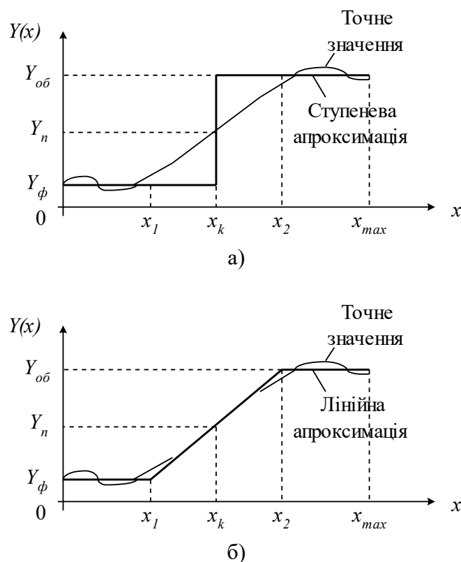
Рисунок 4.1 – Одновимірний перепад яскравості в рядку відеозображення:
