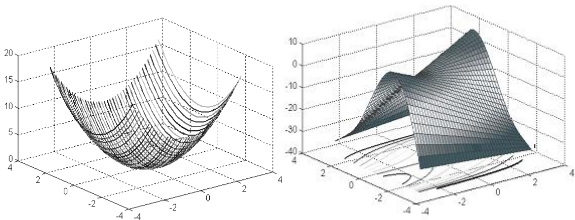
Рис.8.1. Графіки функцій z(x,y)=x^2+y^2 та g(x,y)=5x \cdot \sin x - 3,5y^2
