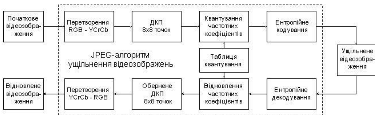
Рисунок 2.1 – Схема JPEG-алгоритму стиснення цифрових відеозображень
