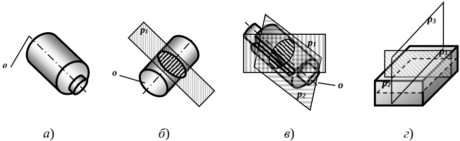
Рис. 10.1.4. Приклади ОВ з різними варіантами взаємного розташування осей обертання та площин симетрії
