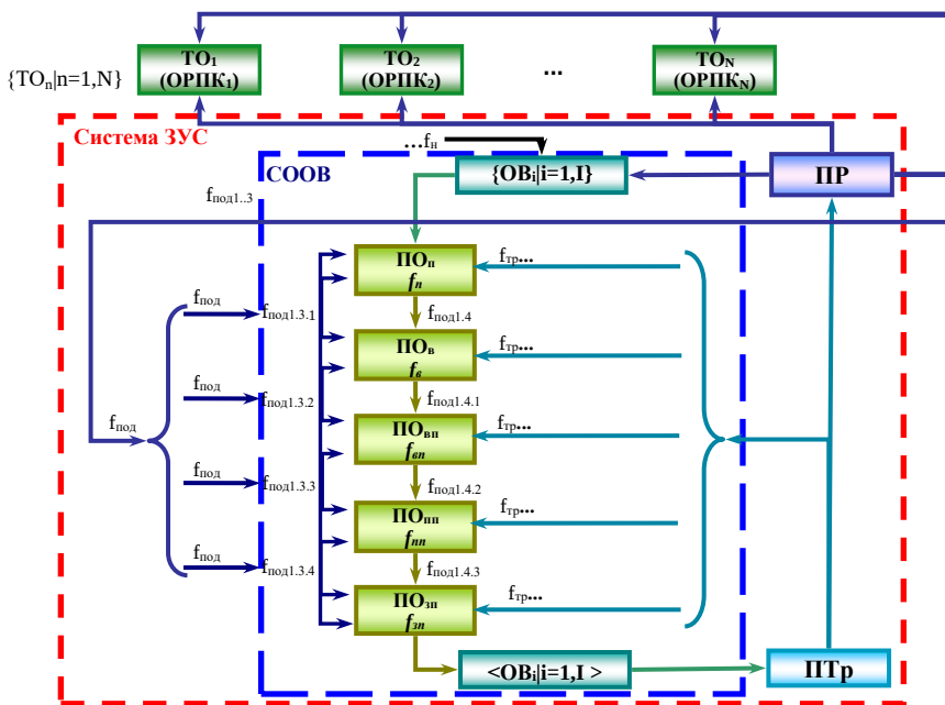
Рис. 10.1.2. Структурна схема ГВС із розвинуеною системою засобів упорядкування середовища (ЗУС):
