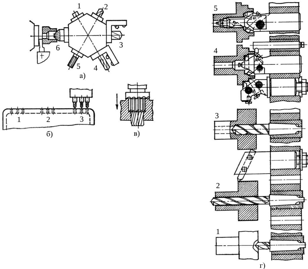
Рис. 4.5. Схема одномісної паралельно-послідовної багатоінструментної обробки: а – на токарно-револьверному верстаті із 6-типозиційною РГ; б – на свердлильному верстаті з послідовним переміщенням (обертанням) багатошпиндельної головки в позиції 1-3-6; в – на свердлильному верстаті комбінованим інструментом; г – на токарно-револьверному верстаті з горизонтальною віссю РГ, наприклад, на верстаті мод. 1Г340ПЦ
