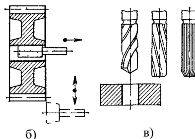
Рис. 4.2. Схеми одномісної послідовної багатоінструментної обробки змінними інструментами: а – токарна обробка зовнішніх циліндричних поверхонь; б – шліфування торця та внутрішньої циліндричної поверхні; в – внутрішньої циліндричної поверхні стрижневими мірними інструментами – свердлом, зенкером, розверткою
