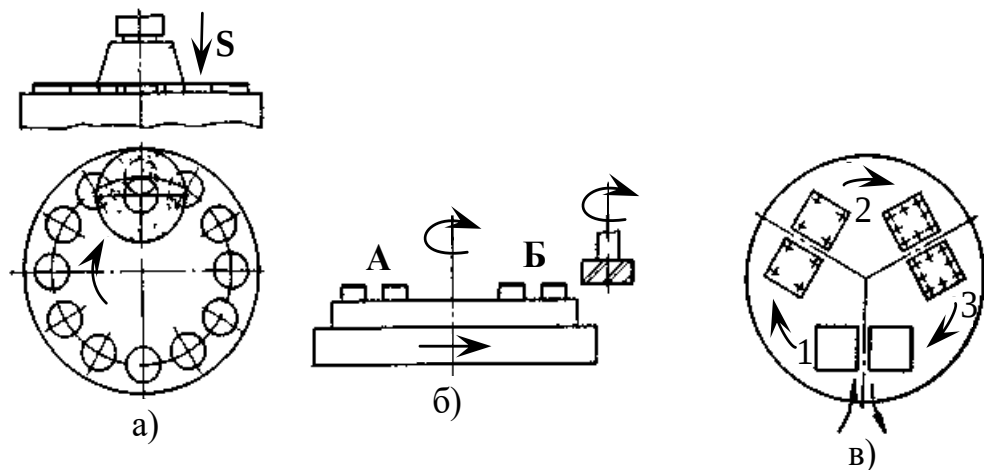
Рис. 4.9. Схеми багатомісної паралельно-послідовної обробки з одночасним (а) і розділним (б, в) встановленням заготовок:
