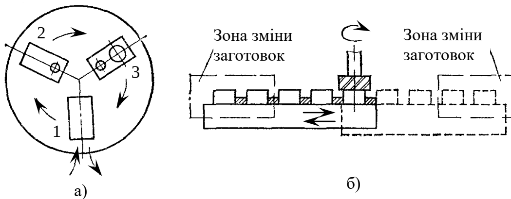
Рис. 4.7. Схеми багатомісної послідовної одноінструментної обробки з роздільним встановленням заготовок:
