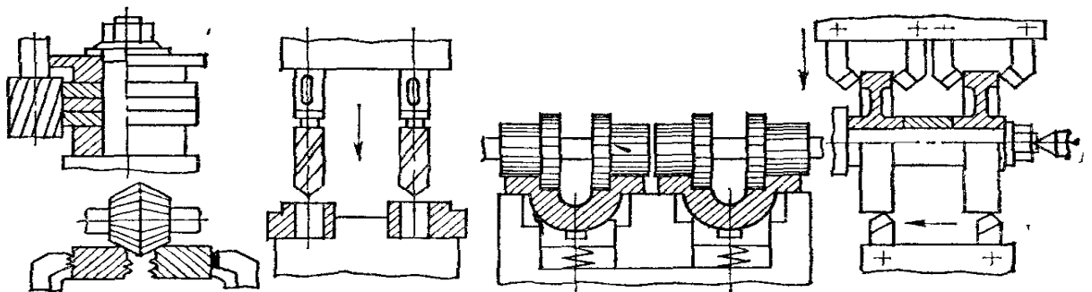
Рис. 4.8. Схеми багатомісної паралельної багатоінструментної обробки з одночасним встановленням заготовок
