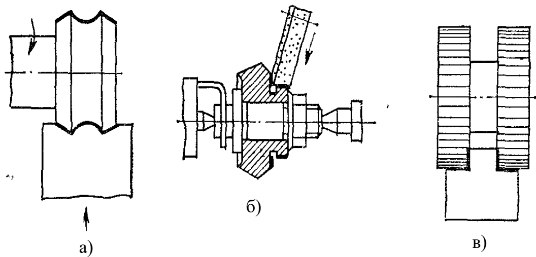
Рис. 4.3. Схема одномісної паралельної одноінструментної обробки: а, б – фасонними інструментами; в – наборами інструментів
