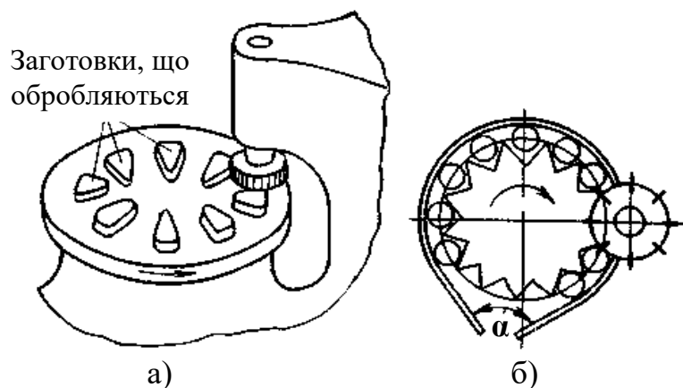
Рис. 4.10. Схеми багатомісної паралельно-послідовної обробки з безперивною зміною заготовок:
