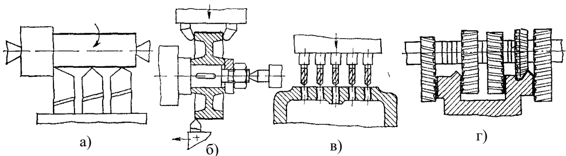
Рис. 4.4. Схеми одномісної паралельної багатоінструментної обробки: а – точіння зовнішньої циліндричної поверхні трома різцями; б – точіння торців та зовнішньої циліндричної поверхні в деталі типу шківів; в – свердлування групи отворів; г – фрезерування поверхонь базової деталі набором фрез
