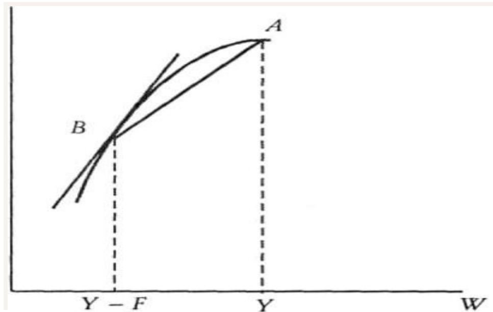
Рис. 1. Залежність очікуваної корисності злочинця від тяжкості та ймовірності покарання
