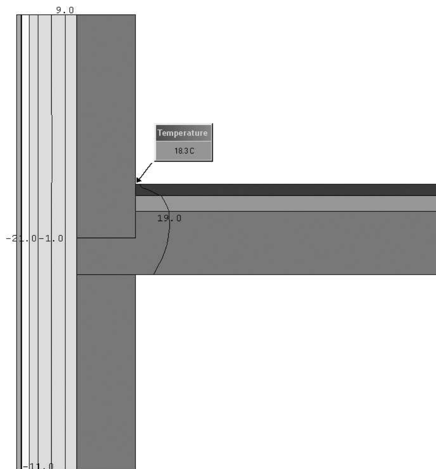
Рисунок А.3 – Температурне поле конструктивного рішення вузла примикання зовнішніх стін до плити перекриття
