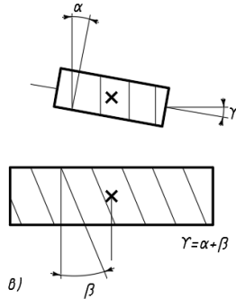
Рис. 3.3. Схеми взаємного розташування фрези на оправці та салазок фрезерного супорта
