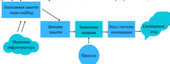
Рис. 07.13. Архітектура Snort
