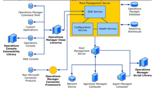
Рис. 07.10 Архітектура SCOM
