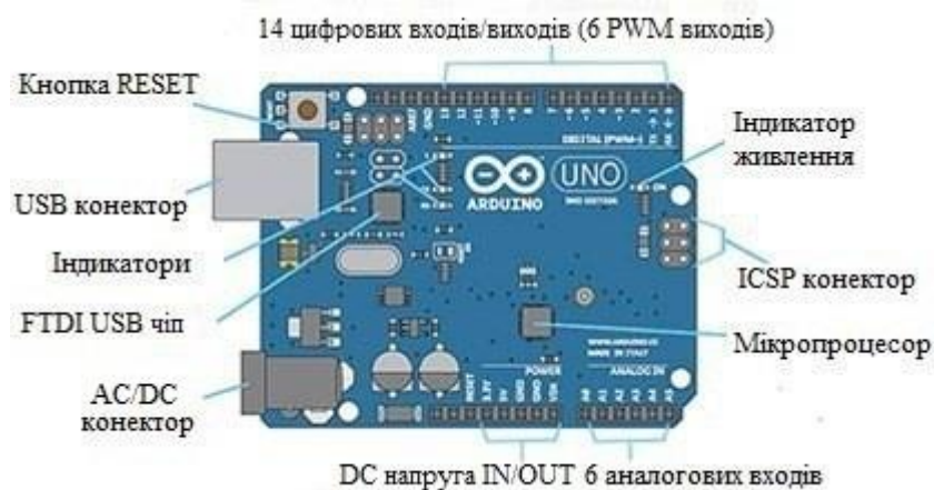
Рис. 2.10. – Контролер Arduino Uno
