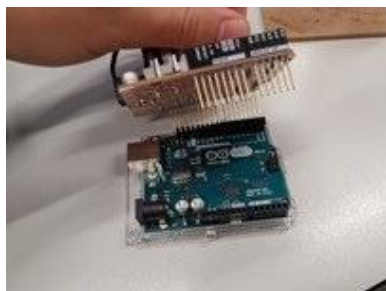
Рис. 2.6. – Загальний вигляд мікроконтролера Arduino Uno та модуля Braccio Shield (а), під'єднання модуля Braccio Shield до Arduino Uno (б), з'єднані модуль Braccio Shield та Arduino Uno (в)
