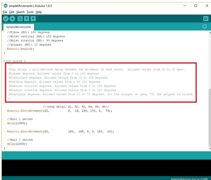
Рис. 2.28. – Приклад простого коду для робота
