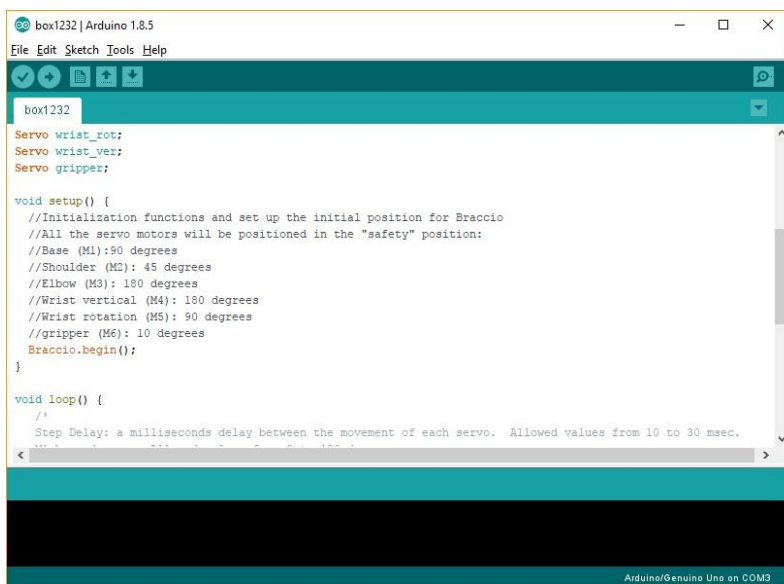
Рис. 2.11. – Вікно середовища розробки програм Arduino IDE
