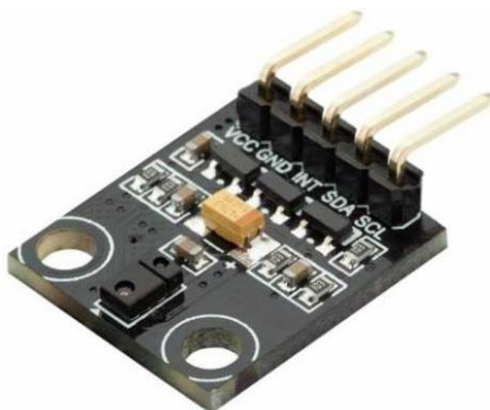
Рис. 3.2. – Зовнішній вигляд датчика кольору RobotDyn APDS-9960
