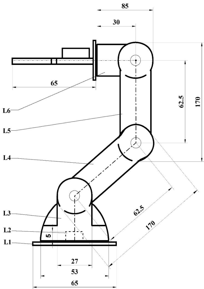
Рис. 2.3. – Основні розміри робота TinkerKit Braccio
