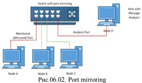
Рис.06.02. Port mirroring
