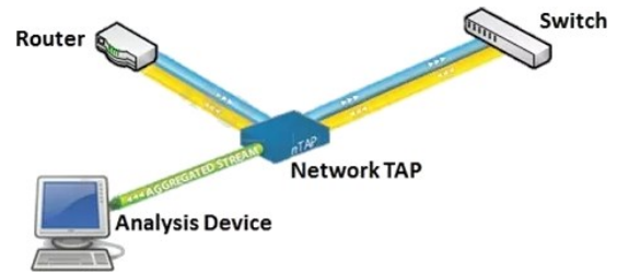
Рис.06.03. Network tap
