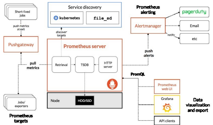
Рис. 05.05. Архітектура Prometheus і деякі компоненти його екосистеми.
