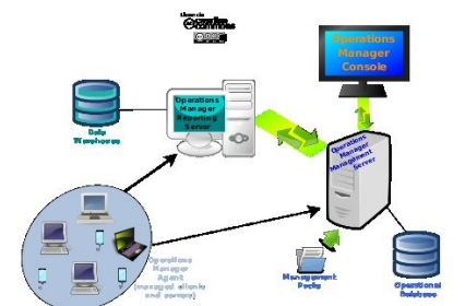
Рис. 05.07. System Center Operations Manager: основні компоненти продукту.
