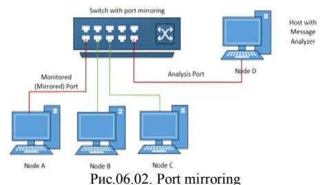
Рис.06.02. Port mirroring
