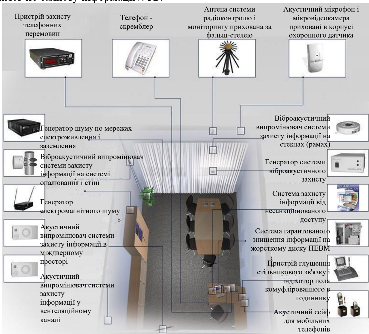
Рисунок 8.1. – Схема комплексу рішень по захисту кімнат переговорів, кабінетів керівників, службових приміщень від просочування конфіденційної інформації по технічних каналах
