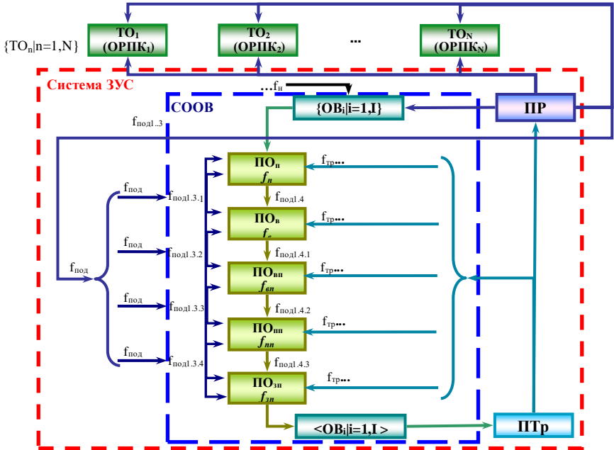
Рис. 7.1.2. Структурна схема ГВС із розвинутою системою засобів упорядкування середовища (ЗУС):
