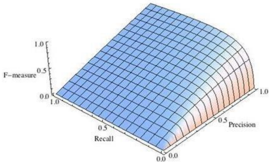
Рис.2 F-міра з пріоритетом точності, \beta^2=1/4
