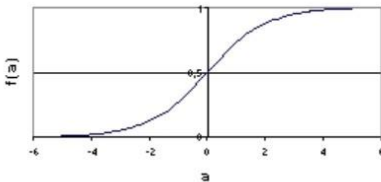
Sigmoide
