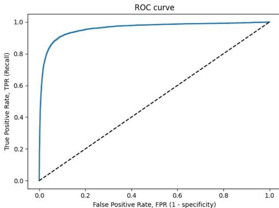
Рисунок 6 –ROC-крива
