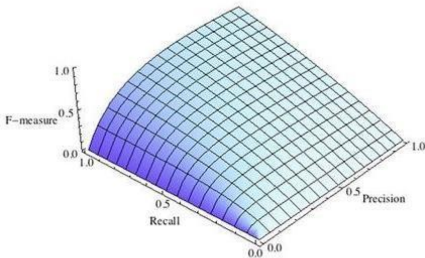
Рис.3 F-міра с пріоритетом повноти, \beta^2=2
