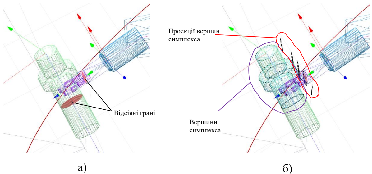
Рис. 7.4. Схема формування множини вершин та їх проєкцій: а) - ілюстрація відсіяних граней; б) вершини симплекса та їх проєкції на одній з відсіяних граней
