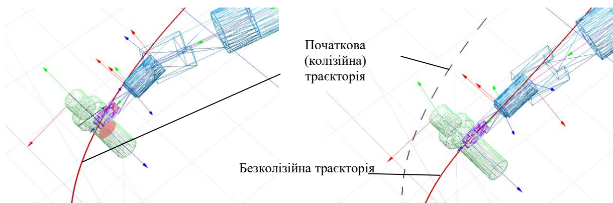
Рис. 7.6. Ілюстрація початкової колізійної та згенерованої безколізійної траєкторії
