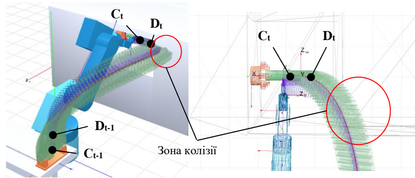
Рис. 7.1. Початкова колізійна траєкторія (зелений тренд)
