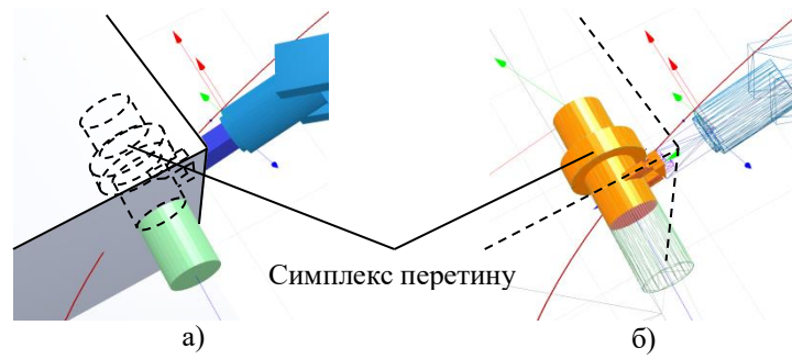
Рис. 7.3. Схема колізійного проникнення ТРК (Сх з ОМ) в перепону: а) загальний вигляд; б) виділена частина проникнення об'ємом V_{colmax}
