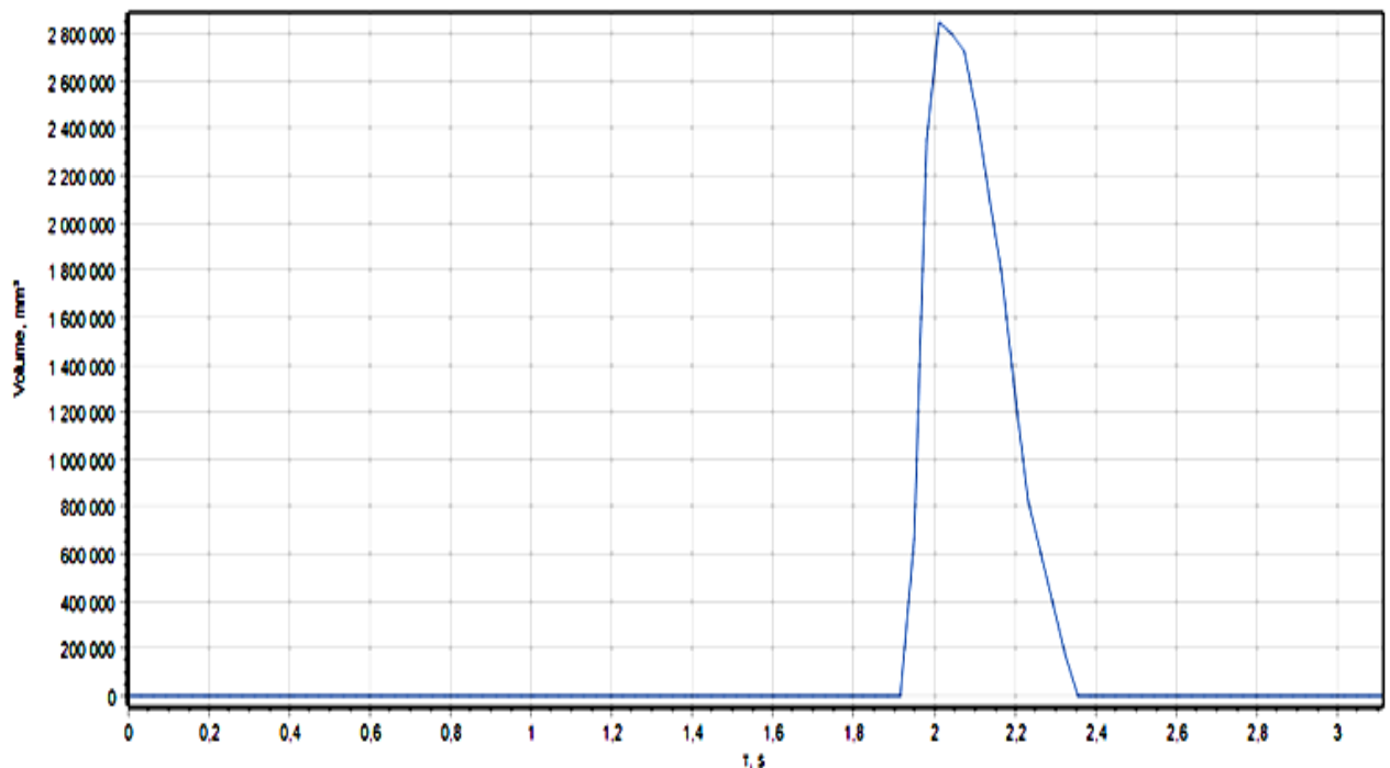
Рис. 7.2. Об'єм і час проникнення ТРК в зоні колізії за рис. 9.1
