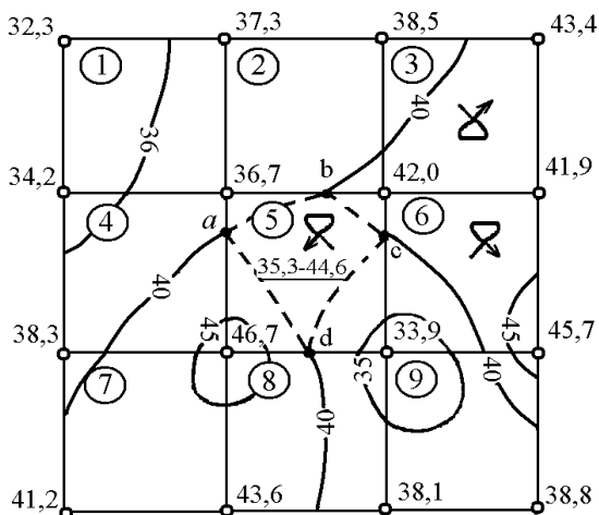
Рис. 25. Побудова плану ізоляції вмісту компонента в руді (за О. Г. Осецьким)
