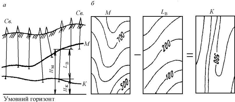
Рис. 5. Схема побудови гіпсометричного плану недостатньо розвіданого пласта К: а – вертикальний розріз; б – віднімання топографічних поверхонь
