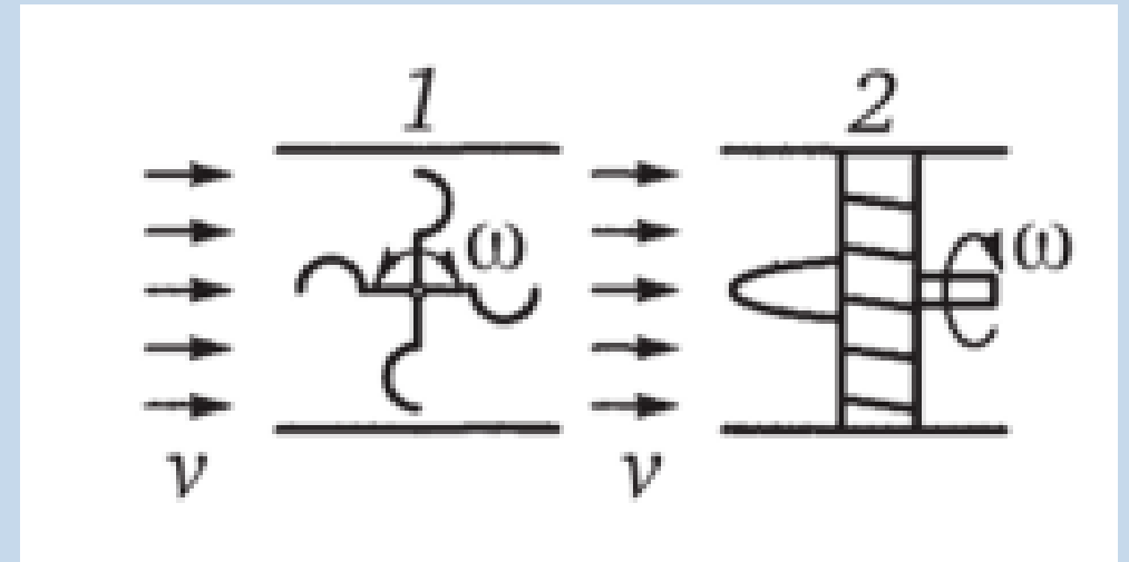
Рис. 4. Турбінний метод: 1 - тангенціальна турбинка; 2 - аксіальна турбинка.
