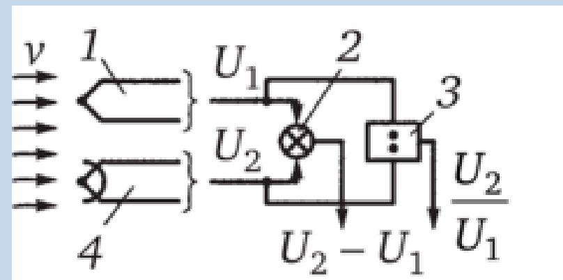
Рис. 3. Термодинамічний метод: 1 - відкрита термопара; 2 - суматор; 3 - дільник; 4 - екранована термопара.
