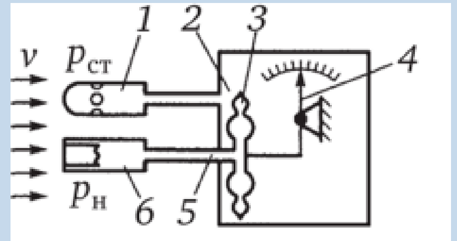
Рис. 1. Аерометричний метод: 1 - приймач статичного тиску; 2 - корпус; 3 - манометрична коробка; 4 - стрілка; 5 - трубопроводи; 6 - приймач повного тиску.
