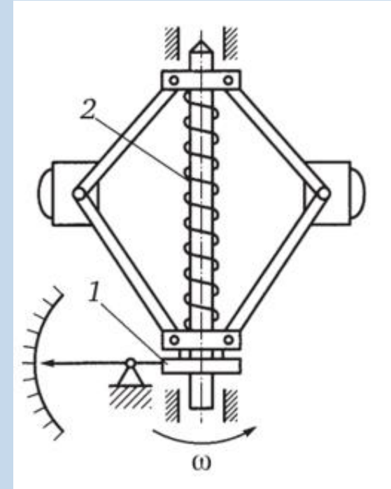
Рис. 5. Конічний тахометр: 1 - муфта; 2 – пружина.
