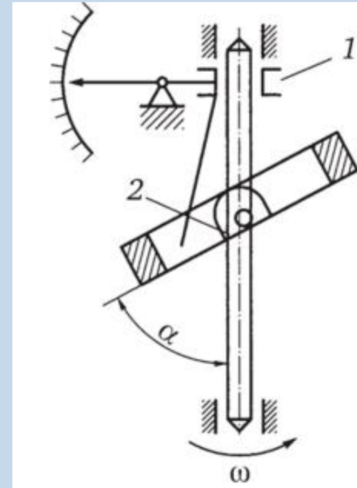
Рис. 6. Кільцевий тахометр: 1 - муфта; 2 - вісь обертання.
