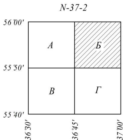
Рис. 5.5. Визначення номенклатури листа карти масштабу 1:50000 (N-37-2-Б)
