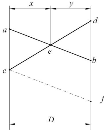
Рис. 4.2. Обчислення відстані від точки нульових робіт до пікета
