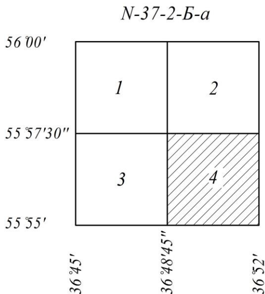
Рис. 5.7. Визначення номенклатури листа карти масштабу 1:10000 (N-37-2-Б-а-4)
