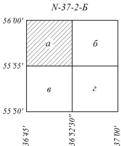
Рис. 5.6. Визначення номенклатури листа карти масштабу 1:25000 (N-37-2-Б-а)
