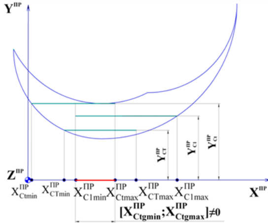
Рис. 11.10. Схема, що ілюструє взаємне розташування множин координат точок \{C_t^{PP} | t = \overline{1, T}\} з непустим перетином [X_{Ctmin}^{PP}; X_{Ctmax}^{PP}] \neq \emptyset
