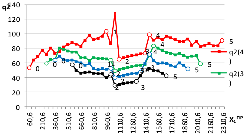
Рис. 11.3. Графіки зміни кінематичного ресурсу q_2 ППР позиційної системи ЧПУ для чотирьох висот ( h_1 - h_4 )
