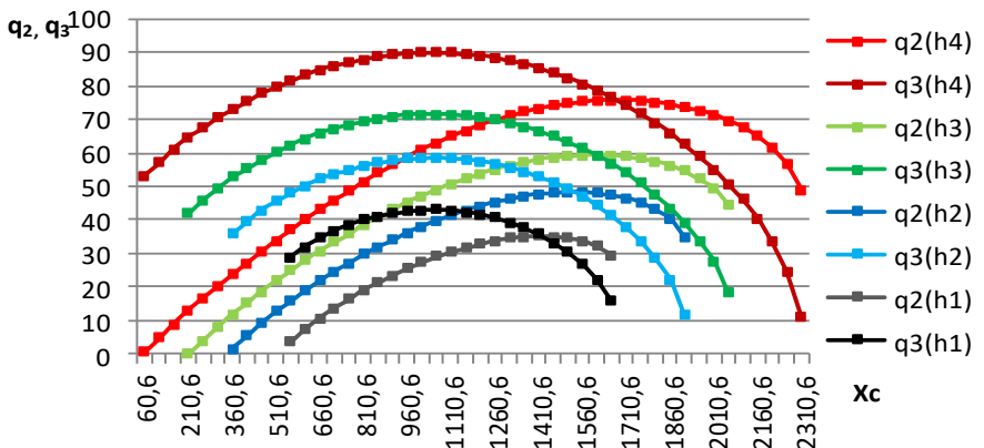
Рис. 11.2. Графіки зміни кінематичного ресурсу ППР контурної системи ЧПУ для чотирьох висот ( h_1 - h_4 )
