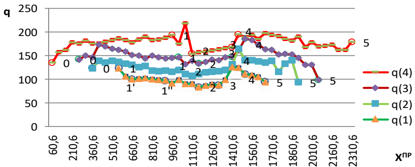
Рис. 11.5. Графіки зміни загального кінематичного ресурсу ППР позиційної системи ЧПУ для чотирьох висот ( h_1 - h_4 )
