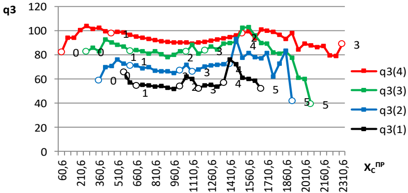
Рис. 11.4. Графіки зміни кінематичного ресурсу q_3 ППР позиційної системи ЧПУ для чотирьох висот ( h_1 - h_4 )
