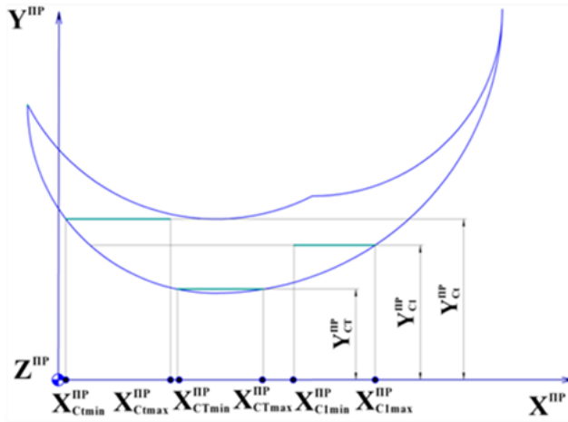
Рис. 11.12. Схема, що ілюструє взаємне розташування множин координат точок \{C_t^{PP} | t = \overline{1, T}\} без перетину (з пустим перетином) [X_{C_{t_{gmin}}^{PP}} ; X_{C_{t_{gmax}}^{PP}}] = 0
