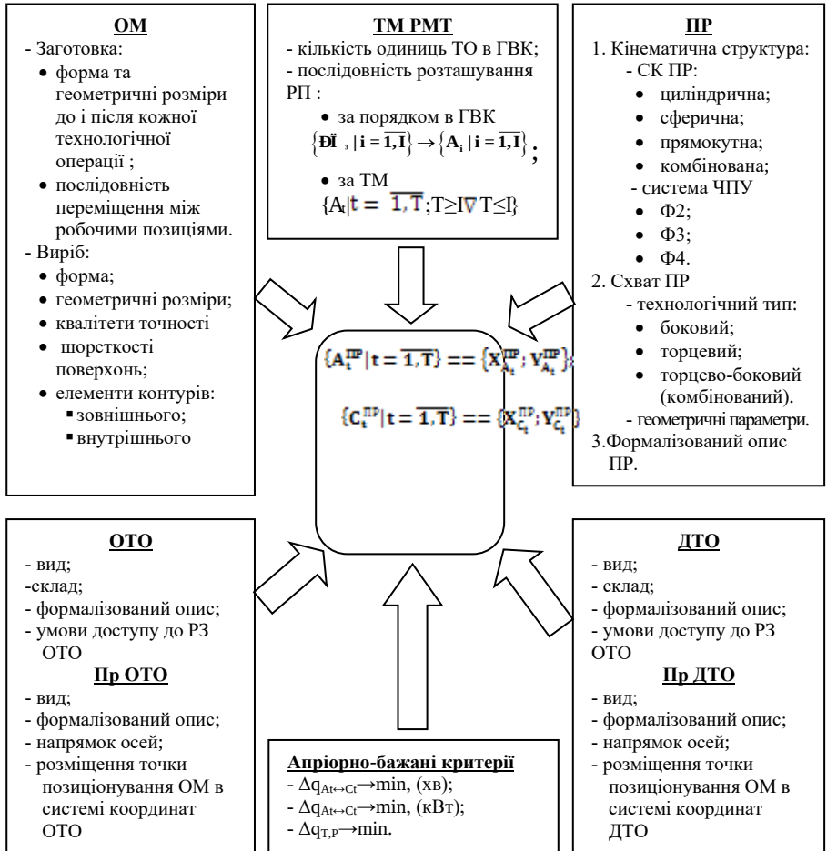
Рис. 11.1. Фактори, що визначають координати опорних точок позиціонування СхПР механоскладальних ГВК
