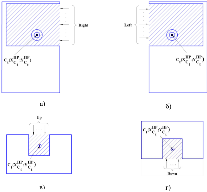
Рис. 11.7. Класифікація закритих ЗО РП: а) закрыта з усіх сторін, крім правої; б) закрыта з усіх сторін, крім лівої; в) закрыта з усіх сторін, крім верху; г) закрыта з усіх сторін, крім низу
