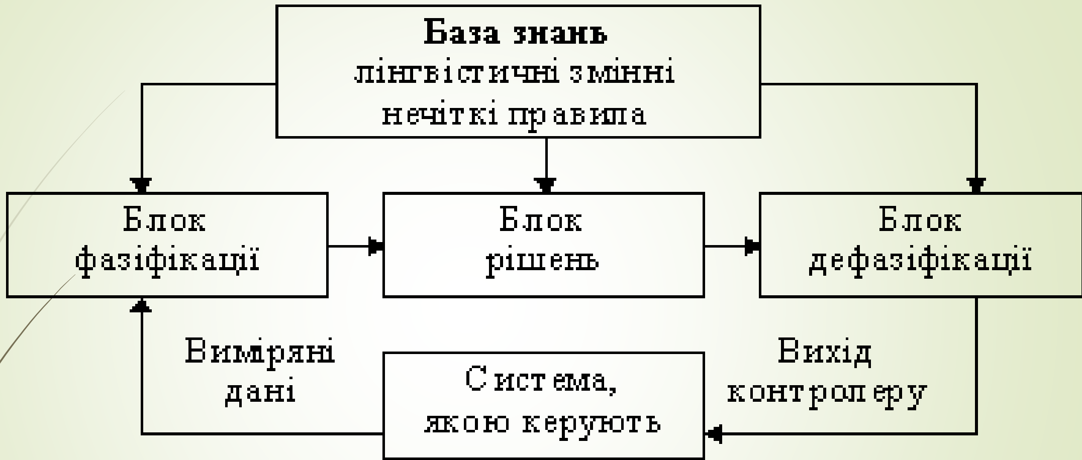
Рис. 1. Загальна структура нечіткого мікроконтролера
