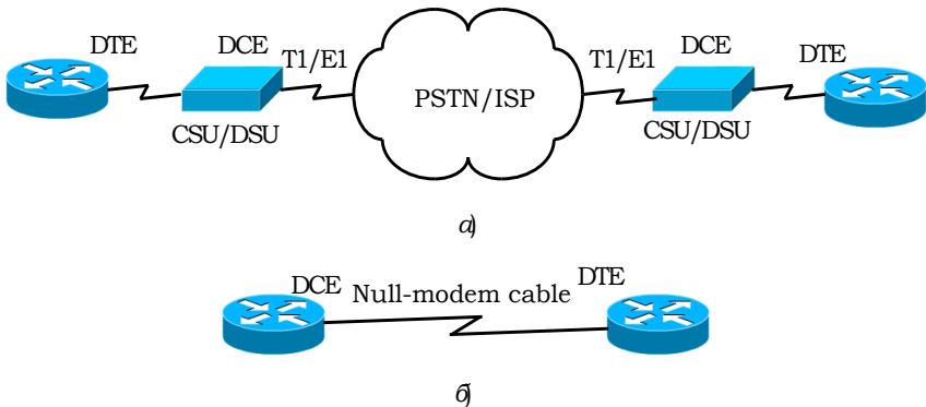
Рис. 5. Підключення за допомогою послідовних інтерфейсів
