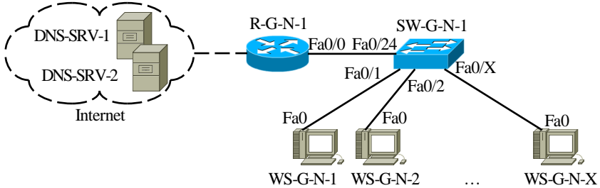
Рис. 27. Проект мережі
