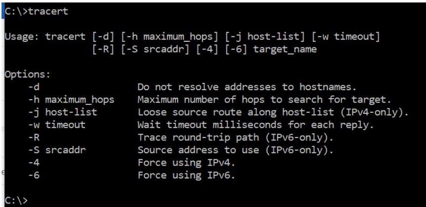
Рис. 6. Перелік ключів(параметрів) команды tracert для ОС Windows 10
