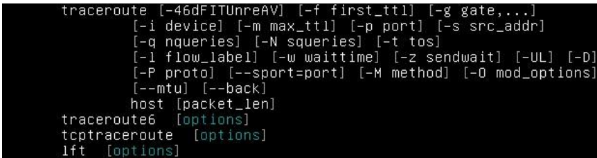
Рис. 5. Перелік ключів(параметрів) команды traceroute для ОС Linux Debian
