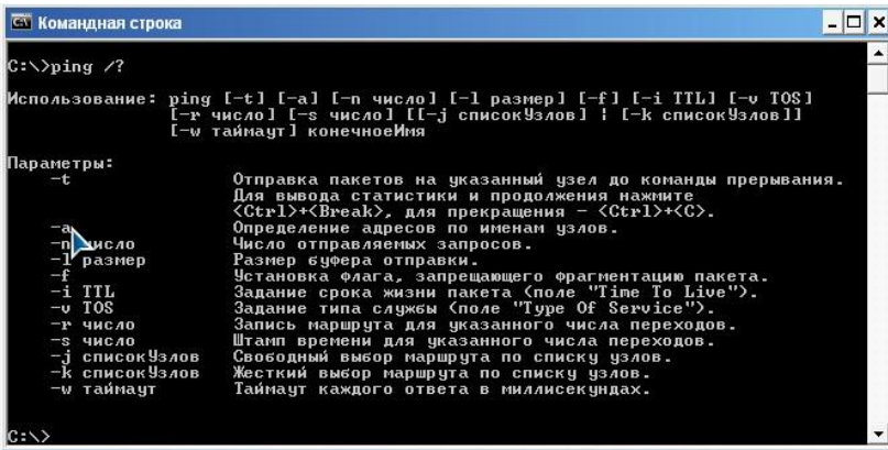
Рис. 1. Перелік ключів(параметрів) команди ping для ОС Windows XP
