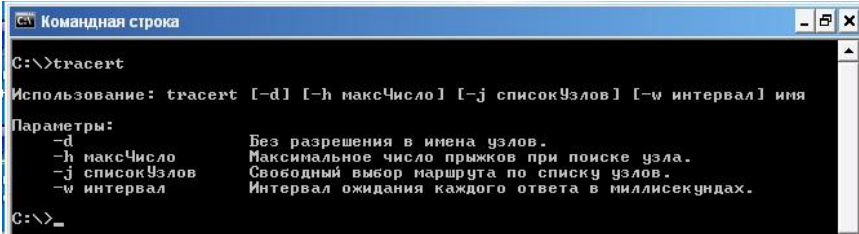
Рис. 4. Перелік ключів(параметрів) команды tracert для ОС Windows XP
