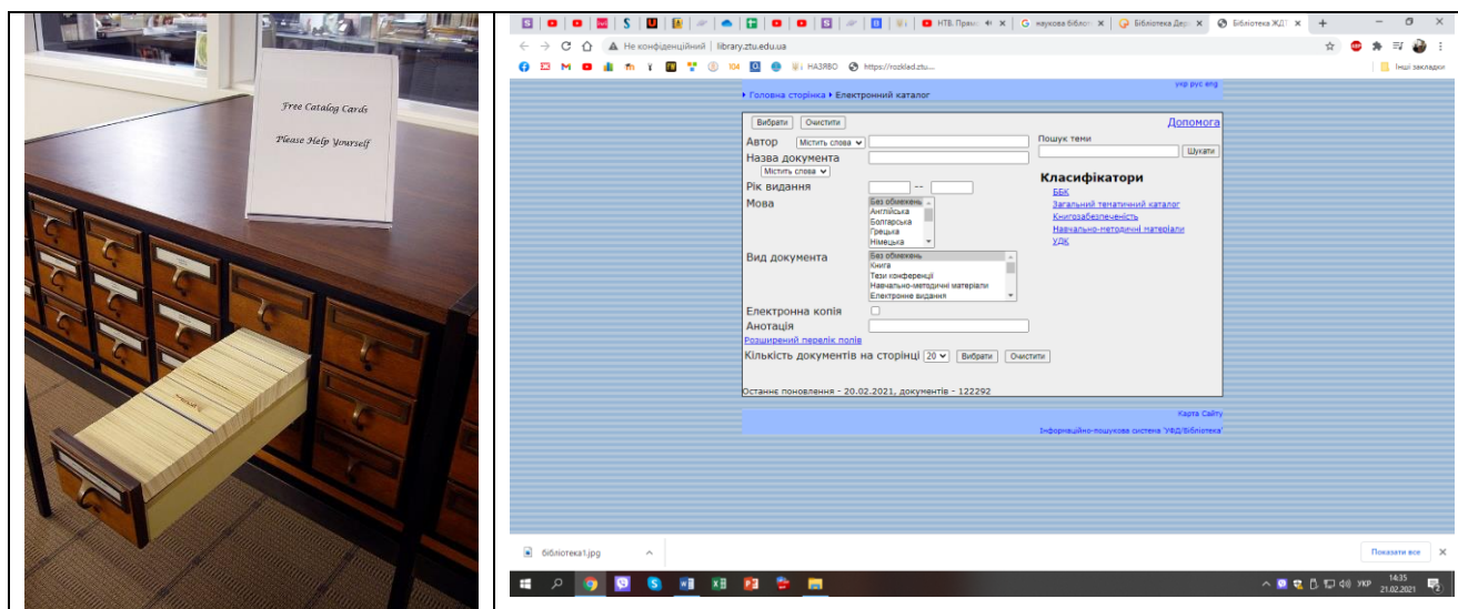
Рис. 1 Бібліотечні каталоги
