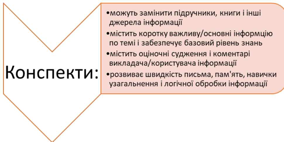
Рис. 1. Функції конспектів
