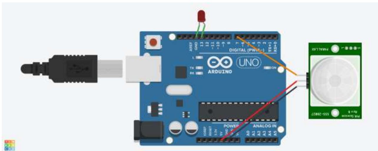
Рисунок 4.3– Схема підключення датчика присутності та світлодіода до Arduino UNO
