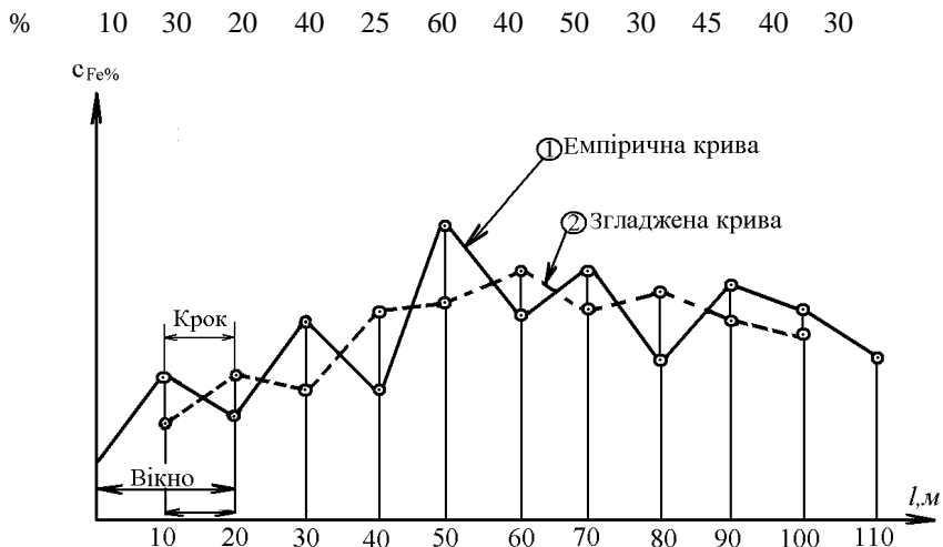
Рис. 15. Згладжування емпіричної кривої методом “ковзного вікна”
