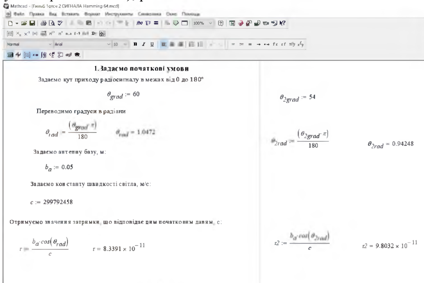
Рис. 4.2 – Початкові умови пеленгування пеленгатора з багатоеlementною лінійною антенною
