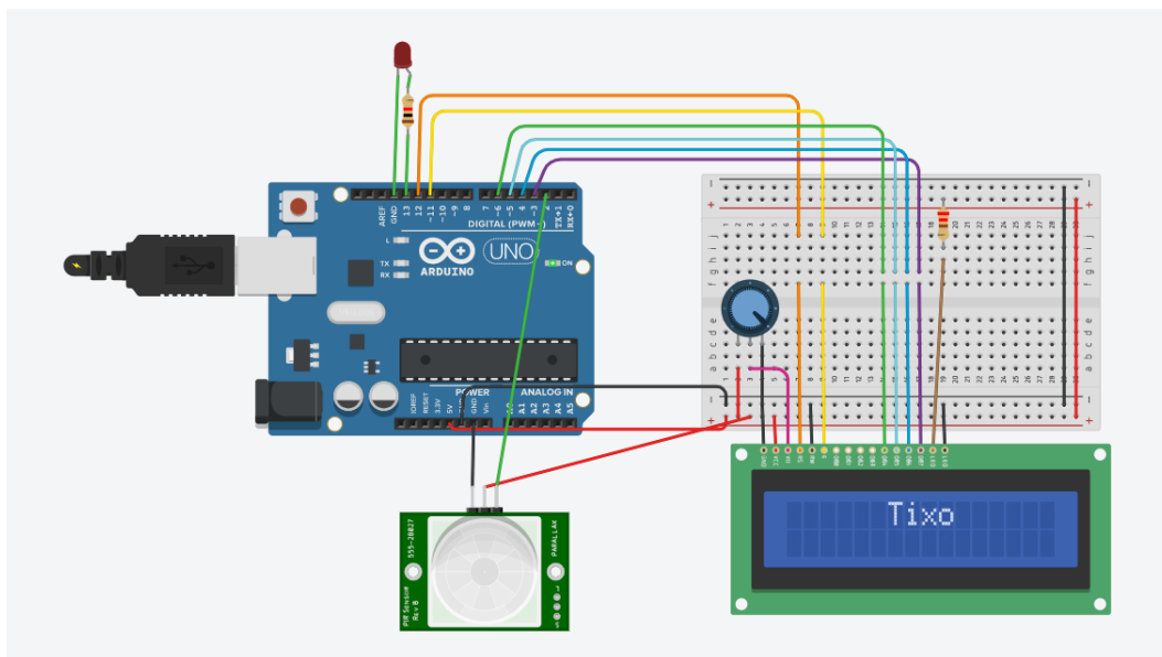
Рисунок 10.3 – Схема підключення датчика присутності та світлодіода до Arduino UNO
