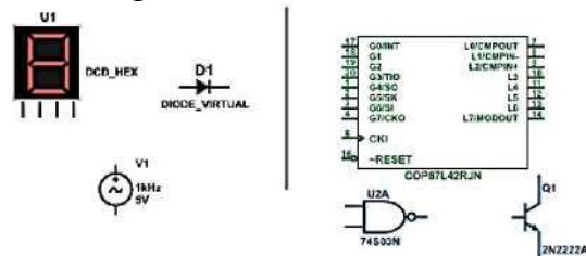
Рис. 10.1. Символи різних компонентів. Віртуальні: 7-сегментний дисплей, діод D1, джерело напруги V1; реальні: логічний елементи HI-I U2A, мікроконтролер U3 і транзистор Q1.
