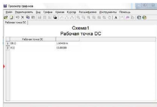
Рис. 11.14. Результат моделювання DC OperatingPointAnalysis
