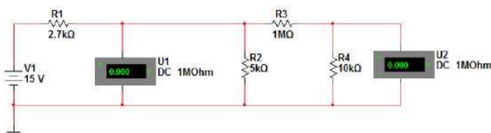
Рис. 11.3. Коло постійного струму з підключеними вольтметрами
