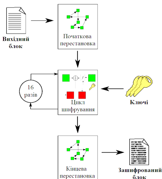
Рис. 3.2. Загальна схема алгоритму DES
