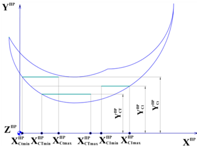
Рис. 10.11. Схема, що ілюструє взаємне розташування множин координат точок \{C_i^{PP} | t = \overline{1, T}\} з частковим перетином [X_{C_{tgmin}}^{PP}; X_{C_{tgmax}}^{PP}] \neq 0
