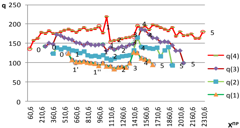
Рис. 10.5. Графіки зміни загального кінематичного ресурсу ППР позиційної системи ЧПУ для чотирьох висот ( h_1 - h_4 )
