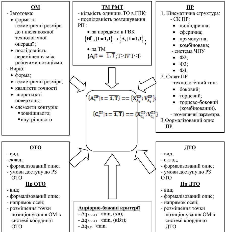
Рис. 10.1. Фактори, що визначають координати опорних точок позиціонування СхРР механоскладальних ГВК
