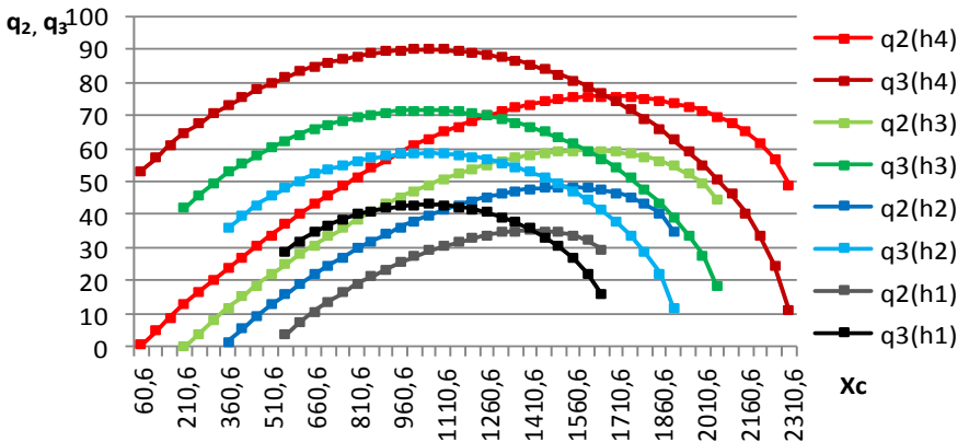
Рис. 10.2. Графіки зміни кінематичного ресурсу ППР контурної системи ЧПУ для чотирьох висот ( h_1 - h_4 )
