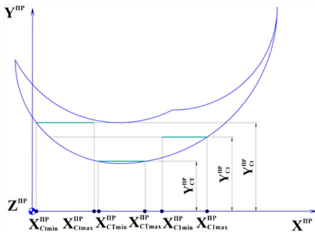
Рис. 10.12. Схема, що ілюструє взаємне розташування множин координат точок \{C_t^{PP} / t = \overline{1, T}\} без перетину (з пустим перетином)
