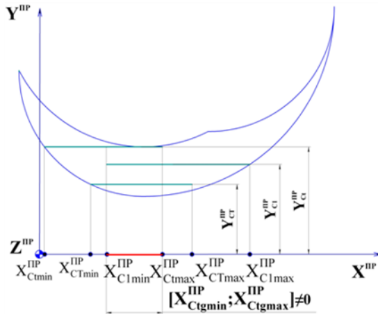
Рис. 9.10. Схема, що ілюструє взаємне розташування множин координат точок \{C_i^{PP} | t = \overline{1, T}\} з непустим перетином [X_{C_{tgmin}}^{PP}; X_{C_{tgmax}}^{PP}] \neq 0
