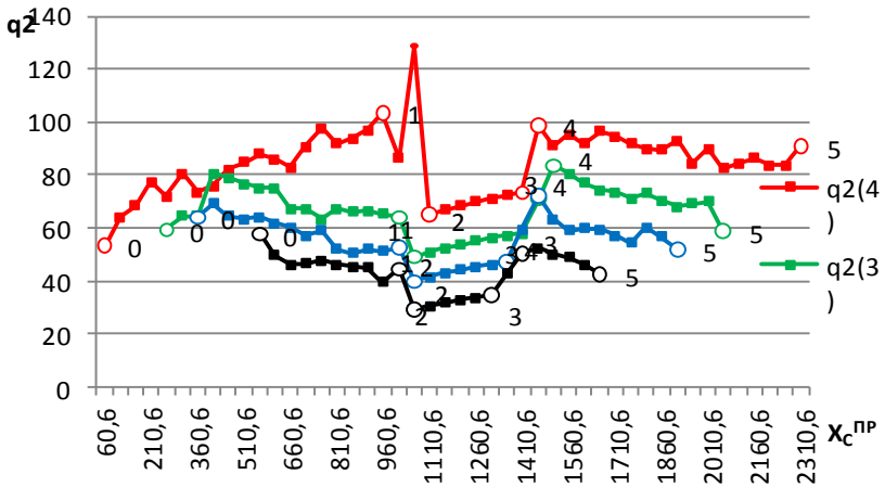
Рис. 10.3. Графіки зміни кінематичного ресурсу q_2 ППР позиційної системи ЧПУ для чотирьох висот ( h_1 - h_4 )
