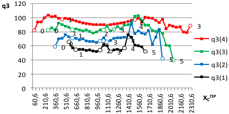
Рис. 9.4. Графіки зміни кінематичного ресурсу q_3 ППР позиційної системи ЧПУ для чотирьох висот ( h_1 - h_4 )
