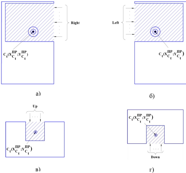
Рис. 10.7. Класифікація закритих ЗО РП: а) закрыта з усіх сторін, крім правої; б) закрыта з усіх сторін, крім лівої; в) закрыта з усіх сторін, крім верху; г) закрыта з усіх сторін, крім низу
