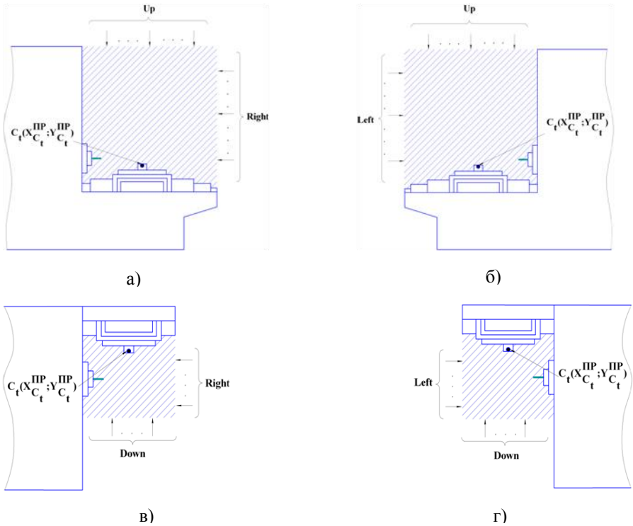
Рис. 10.8. Класифікація напіввідкритих 3О РР:
