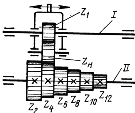
Рис. 6.2. Механізм Нортон
