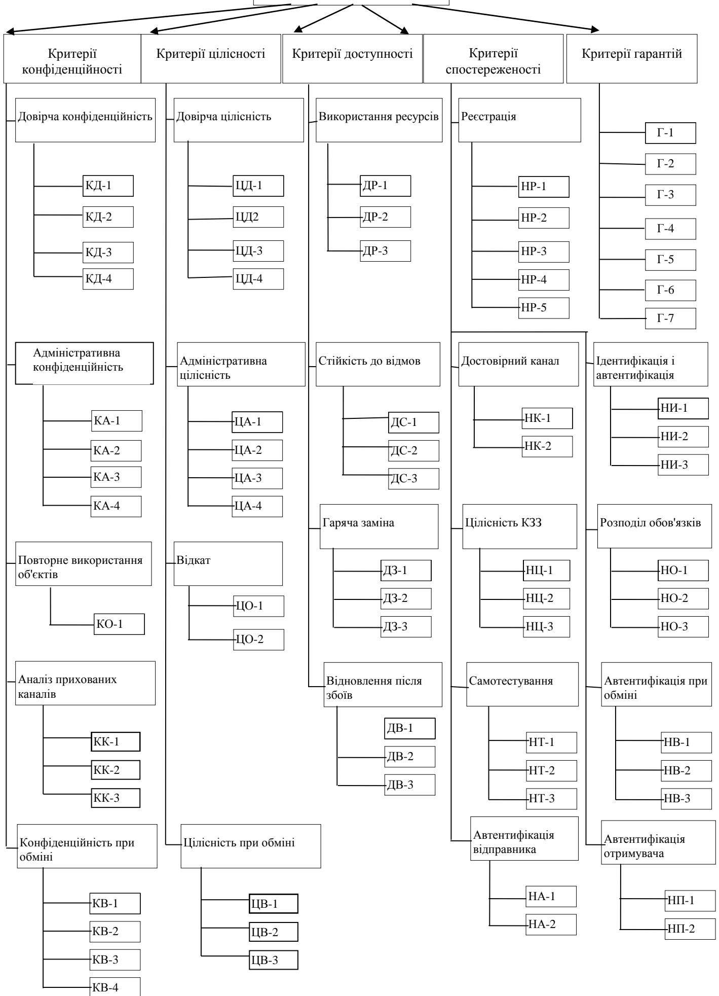
Рисунок 1 - Структура критеріїв
