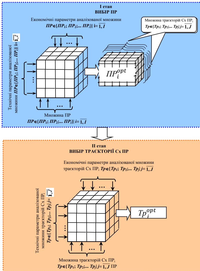
Рис. 10.2. Спрощена схема послідовності вибору ПР та оптимальної траєкторії Сх ПР при синтезі РМСТ
