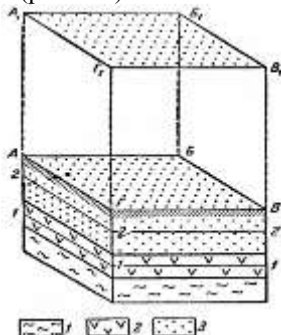
Рис. 7.1. Зображення на геологічній карті горизонтальне залягання пластів в умовах горизонтального рельєфу ABVG – горизонтальна поверхня місцевості; A_1B_1V_1Г_1 – проекція поверхні ABVG на горизонтальну площину (геологічна карта); 1, 2, 3 – горизонтально залягаючі пласти різного складу
