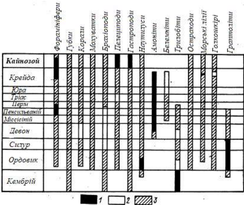
Рис. 2.4. Відносне хроностратиграфічне значення основних груп морських безхребетних протягом геологічного часу
