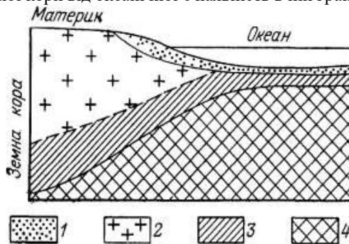
Рис. 1.4. Схема будови континентальної і океанічної кори 1 – осадовий шар; 2 – гранітний шар; 3 – базальтовий шар; 4 – мантія
