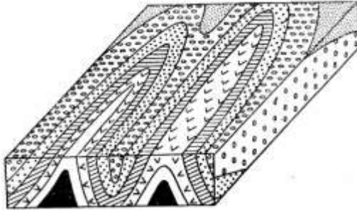
Рис. 7.6. Зображення антиклінальних і синклінальних складок на геологічній карті
