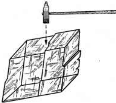
Рис. 3.6. Визначення напрямку спайності в кальциту
