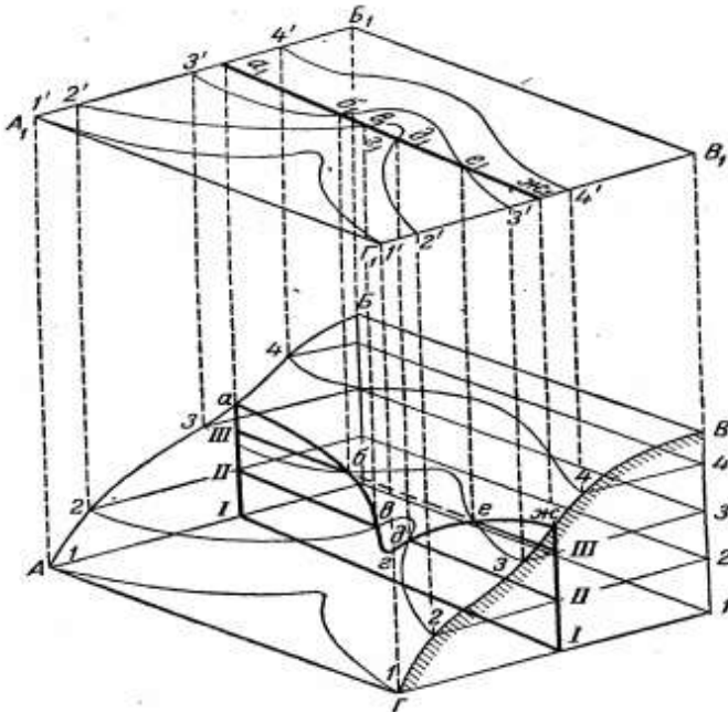
Рис. 7.5. Зображення на геологічній карті вертикально залягаючого пласта
