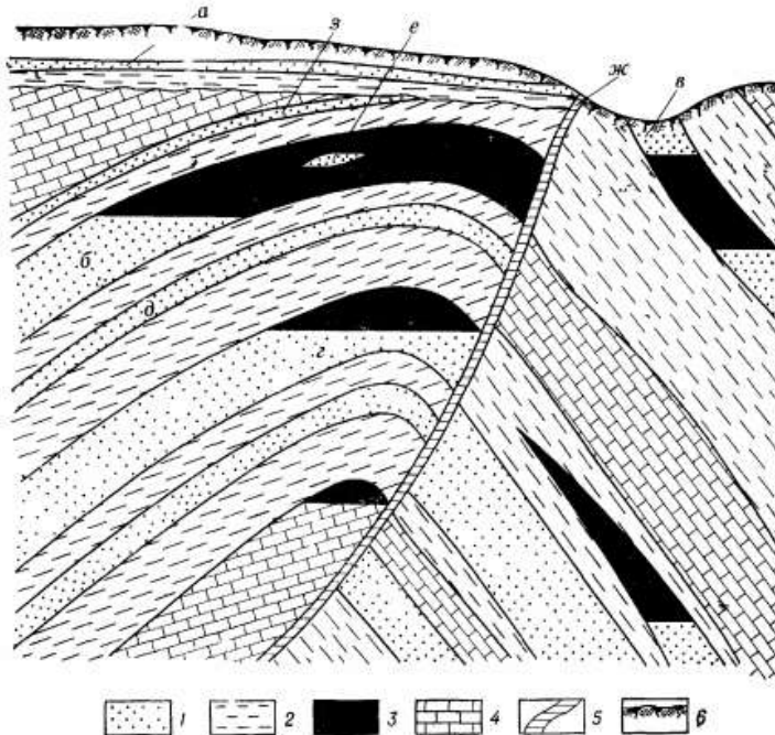
Рис. 8.5. Промислова класифікація підземних вод
