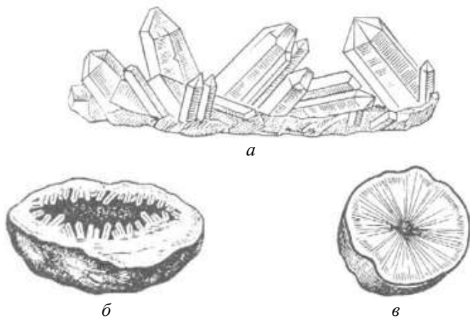
Рис. 3.5. Мінеральні агрегати: a – друзи; б – секреція; в – конкреція
