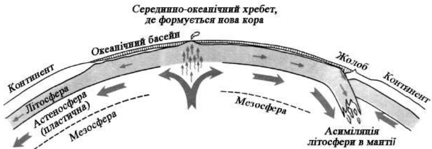
Рис.1.3. Розростання океанічного дна
