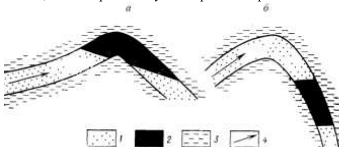
Рис. 8.4. Зміщення покладу нафти рухомими водами а – поклад з нахилом ВНК; б – висячий поклад 1 – водоносний горизонт; 2 – нафтовий поклад; 3 – водотриви; 4 – напрям руху підземних вод
