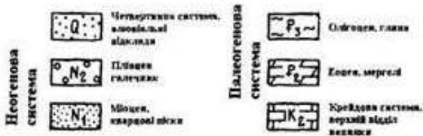
Рис. 7.11. Стратиграфічна колонка
