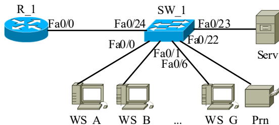
Рис. 2. Приклад мережі
