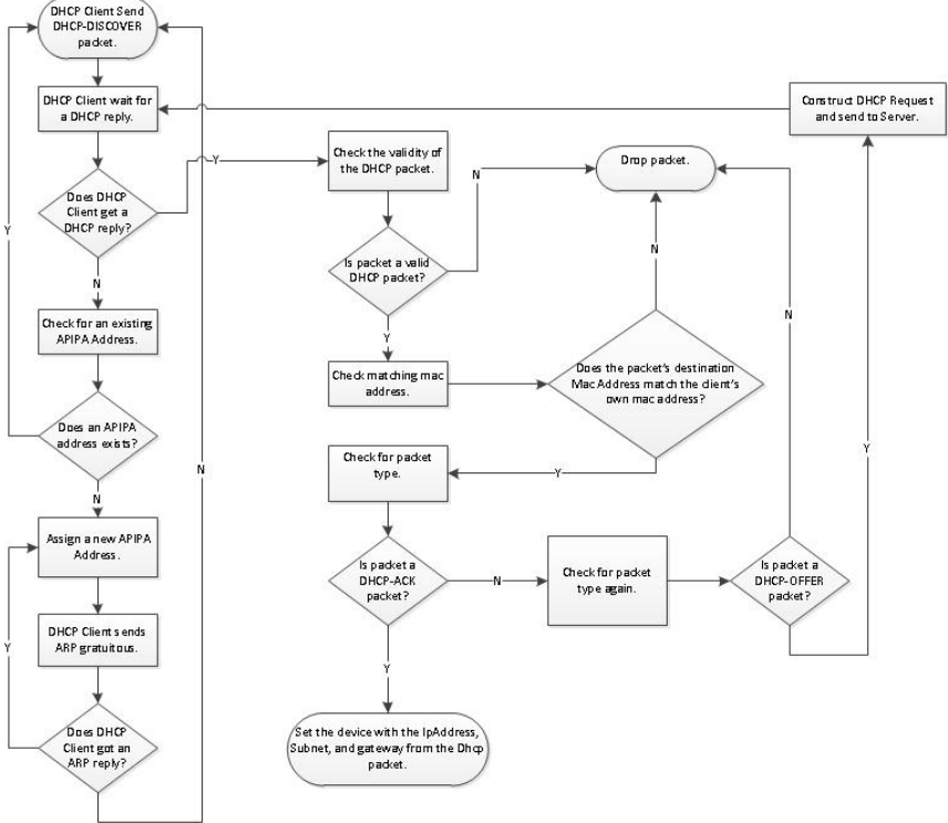
Рис. 1. Блок-схема алгоритму функціонування DHCP-клієнта
