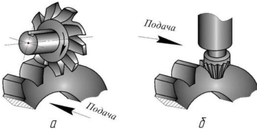
а – дисковою фрезой; б – пальцевою фрезой
