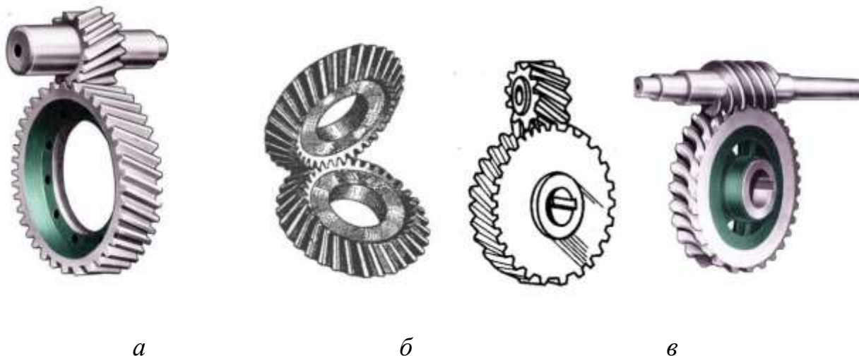
Рисунок 3.3 – По розташуванню осей валів у просторі
