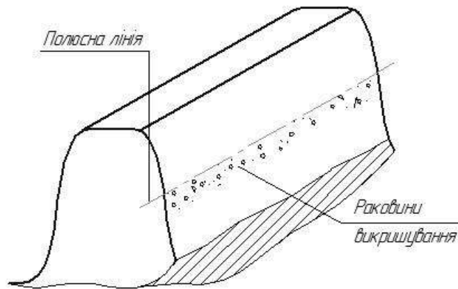
Рисунок 3.10 – Викришування на поверхні ніжок зубців
