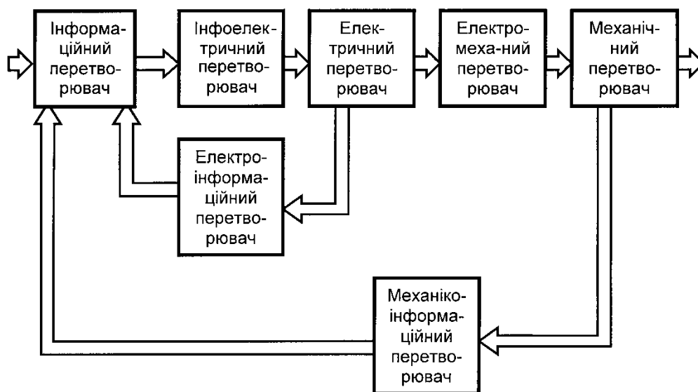
Рис. 4.3. Функціональна модель ( F -модель) МТМ
